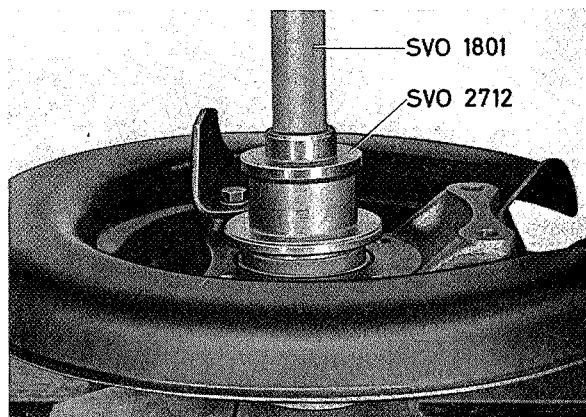
Fig. 4-83. Montage van de buitenste vetkeerring
