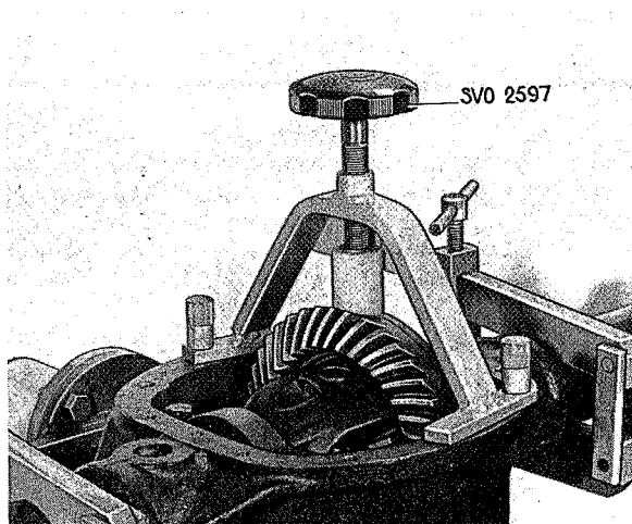
Fig. 4-115. Remgereedschap voor het differentieel
