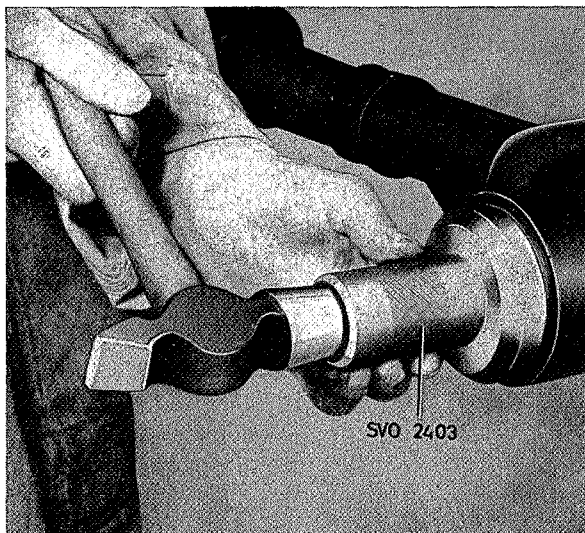
Fig. 4-92. Montage van de oliekeerring
