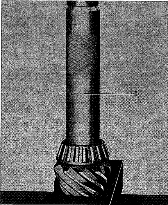
Fig. 4-111. Montage van het achterste pignionlager 1. Montagehuls SVO 2395
