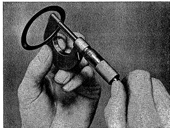
Fig. 4-110. Het meten van de shims
