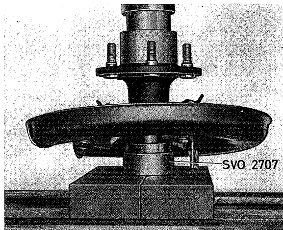
Fig. 4-84. Montage van de aandrijf-as
