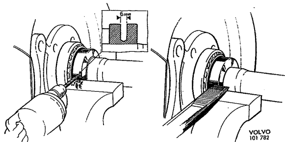
Fig. 4-81. Het verwijderen van de borgring
