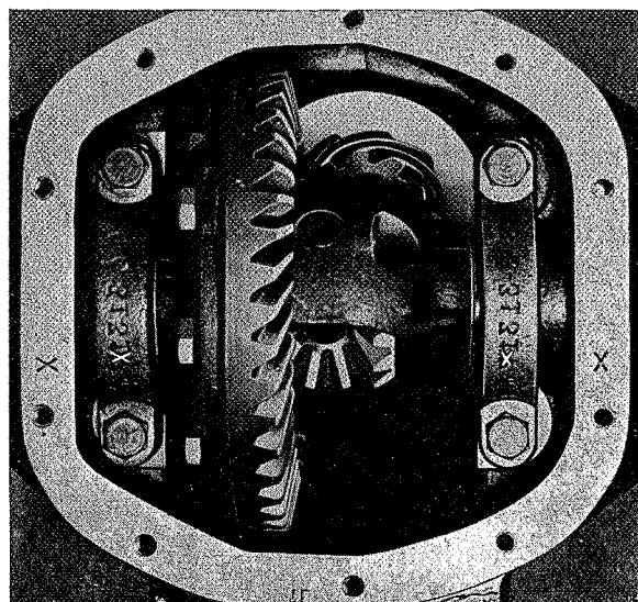
Fig. 4-95. De tekens op kap en huis
