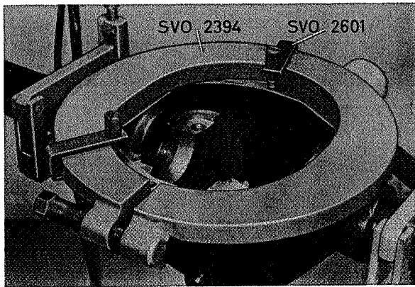
Fig. 4-96. Het uitzetten van het achterashuis
