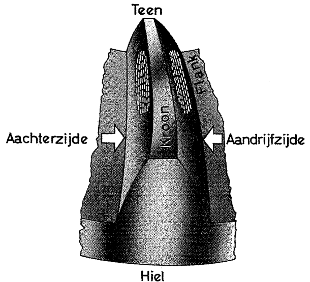
Fig. 4-116. Het juiste tandcontact
