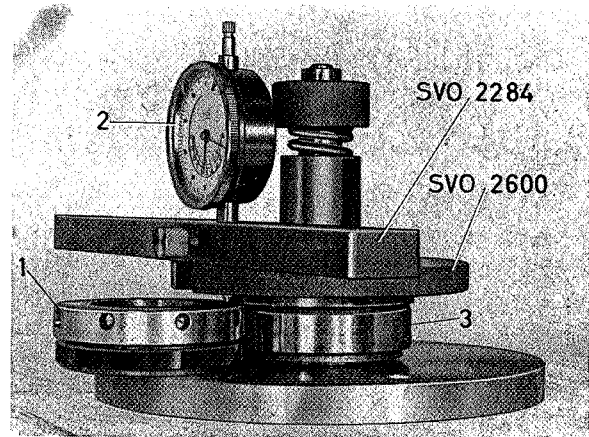
Fig. 4-107. Het vaststellen van de dikte van de shims 1. Afstelring 2. Meetklok 3. Lager, compleet
