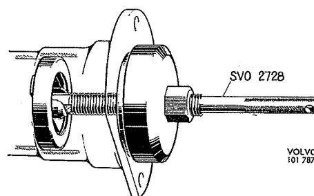
Fig. 4-85. Demontage van de binnenste oliekeerring
