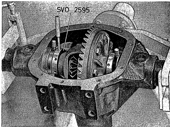
Fig. 4-114. Afstelringen van het differentieelhuis
