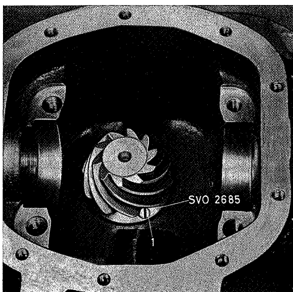
Fig. 4-104. Het afstellen van de pignon met de afstelring 1. Klemschroef
