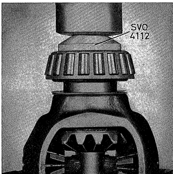
Fig. 4-119. Montage van de differentieellagers
