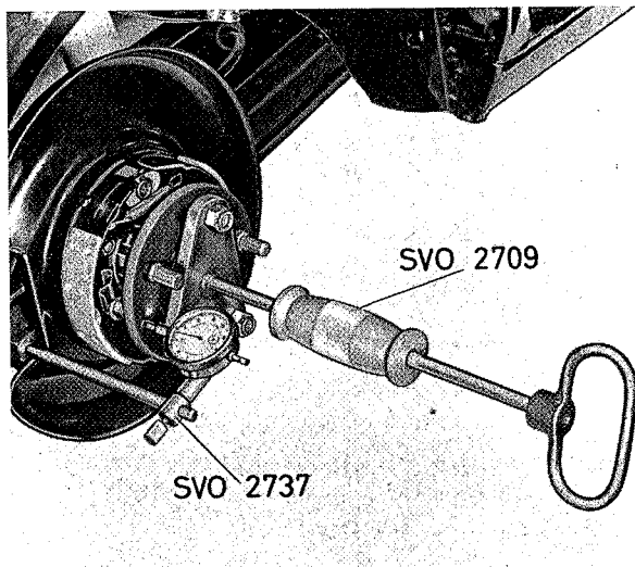
Fig. 4-88. Het meten van de axiale speling van de aandrijfas
