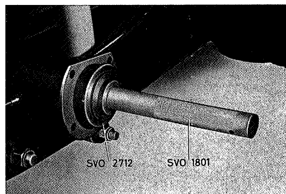
Fig. 4-86. Montage van de binnenste oliekeerring
