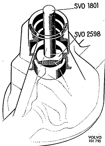
Fig. 4-97. Demontage van de achterste pignoncup
