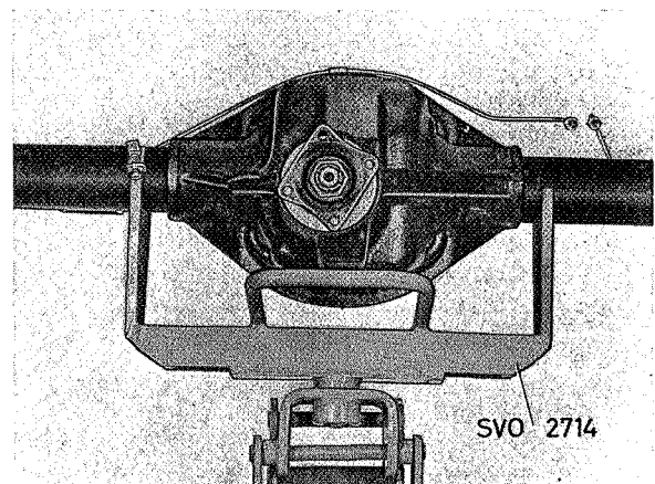
Fig. 4-120. Steun voor de achteras
