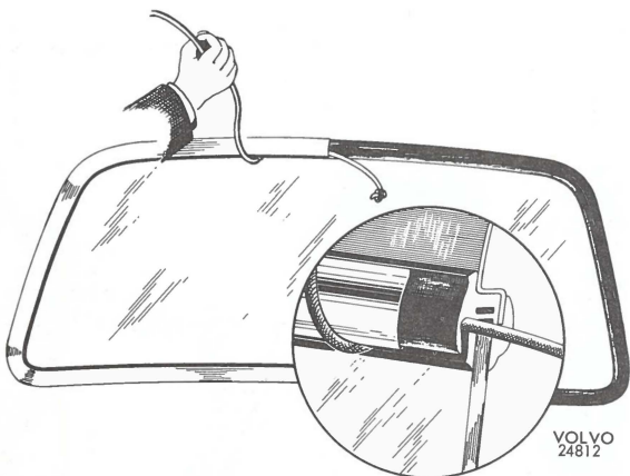
Fig. 7. Inzetten van de ruit
