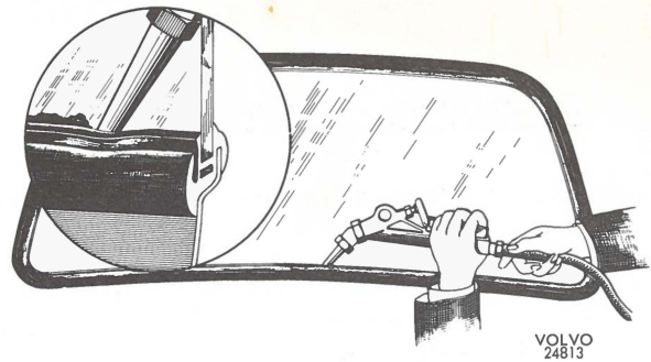
Fig. 8. Afkitten van de ruit
