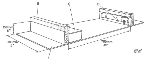
Fig. 10. Bok waarop de ruit wordt gelegd voor het omleggen van het ruitrubber
