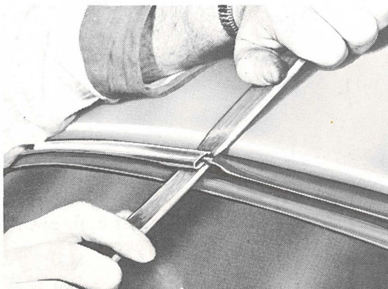
Fig. 2. Loswerken van de sierlijst uit het ruitrubber
