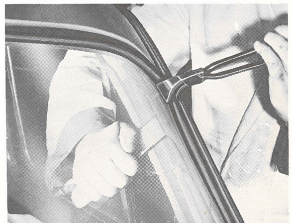
Fig. 4. Lostrekken van het ruitrubber
