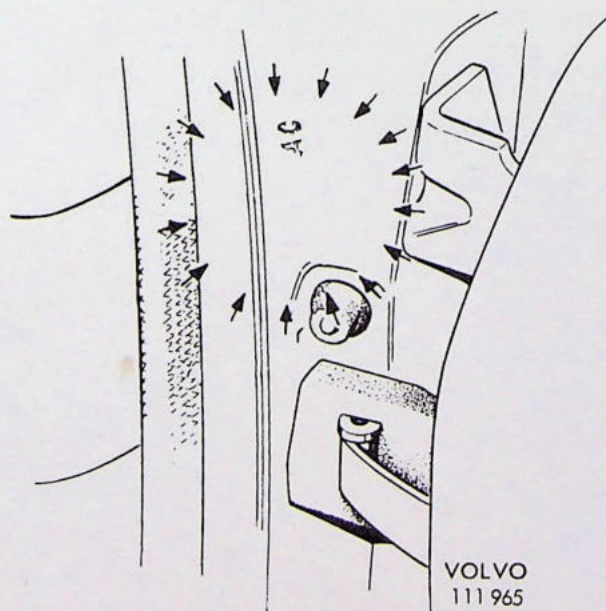
Fig. 1. 164 en de 140 series tot en met het 1972 model, deurstijl, rechterzijde. De code wordt door de pijlen aangegeven.
