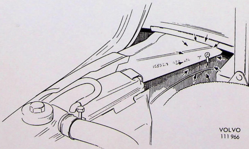
Fig. 3. 1800: Voorste bovenste verbindingbalk rechterzijde.
