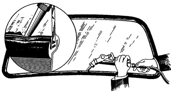
Fig. 8-24. Het aanbrengen van afdichtkit
