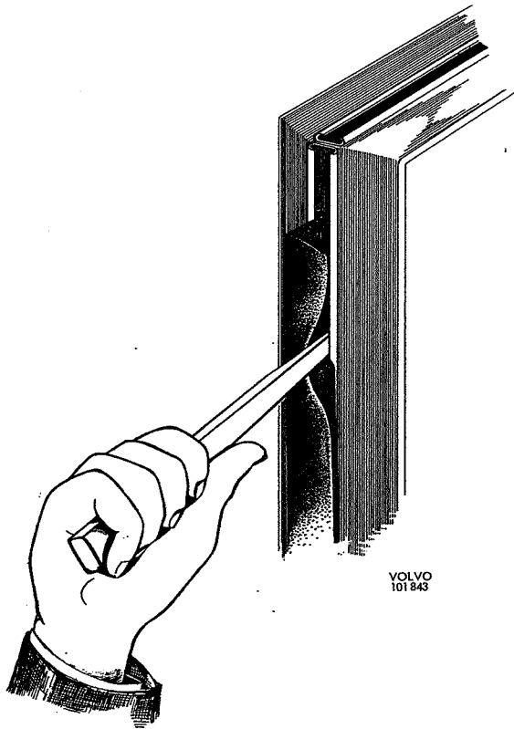
Fig. 8-16. Montage van de afsluitstrook
