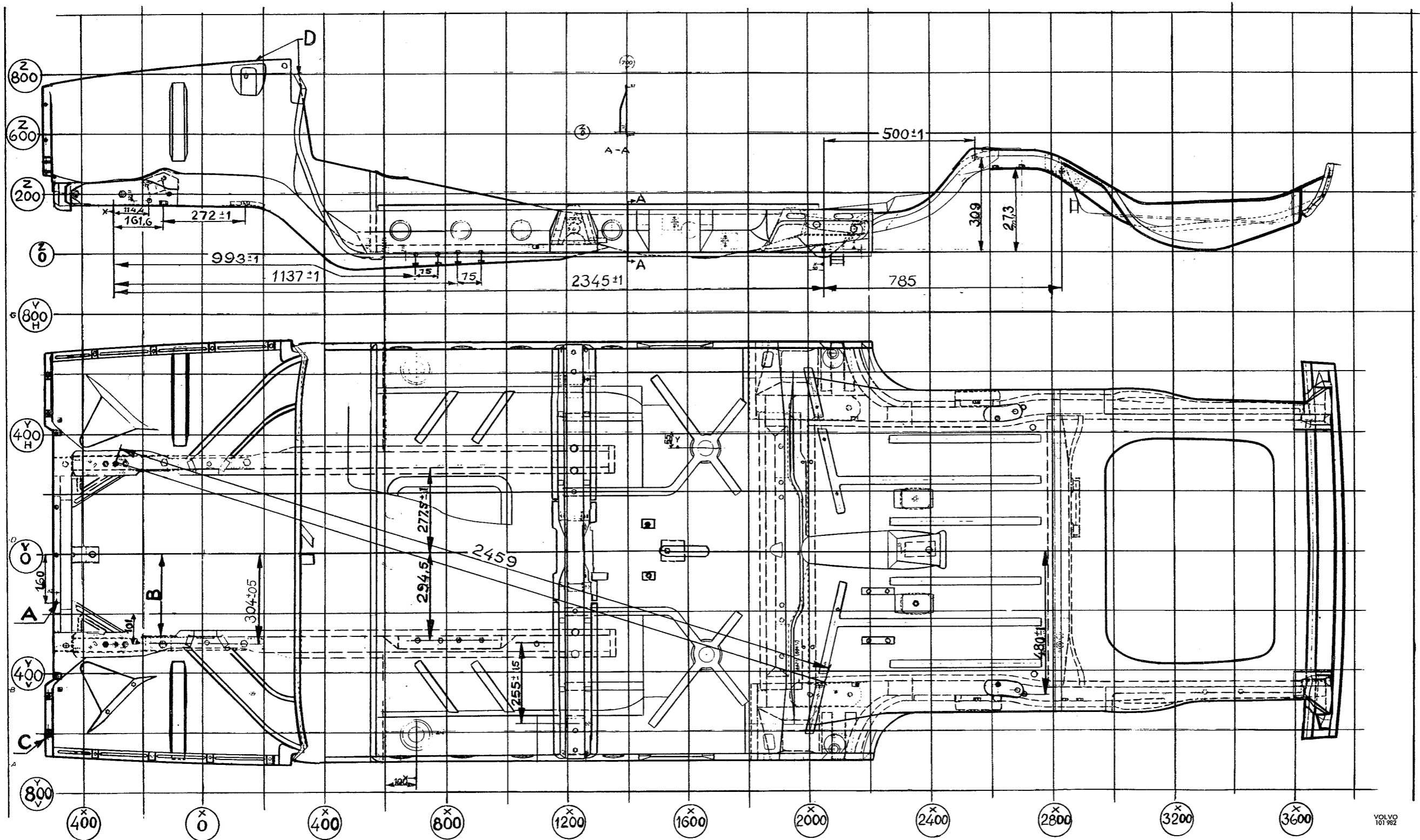
Tekening 8 A. Kontroletekening voor karrosserievloer
