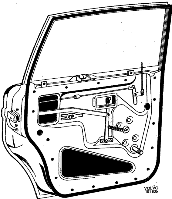
Fig. 8-7. Achterportier
