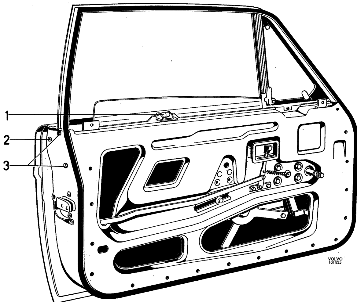
Fig. 8-6. Voorportier
