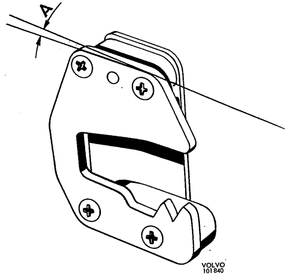
Fig. 8-11. Palplaat A. Voorportier 1,5° Achterportier 2,5°
