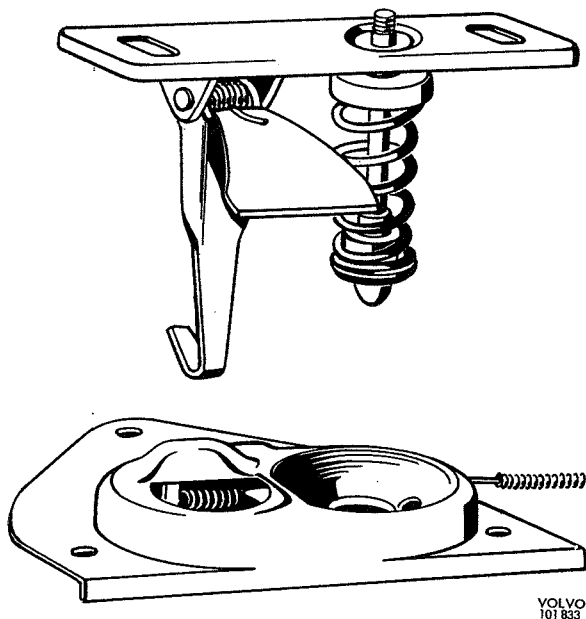
Fig. 8-4. Slot van motorkap
