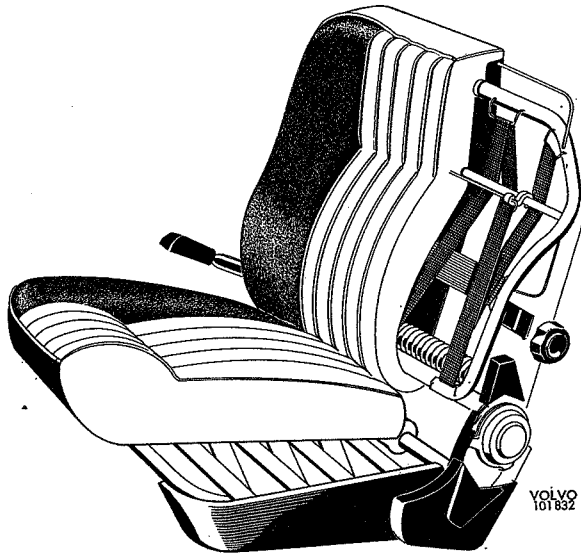
Fig. 8-3. Voorstoel
