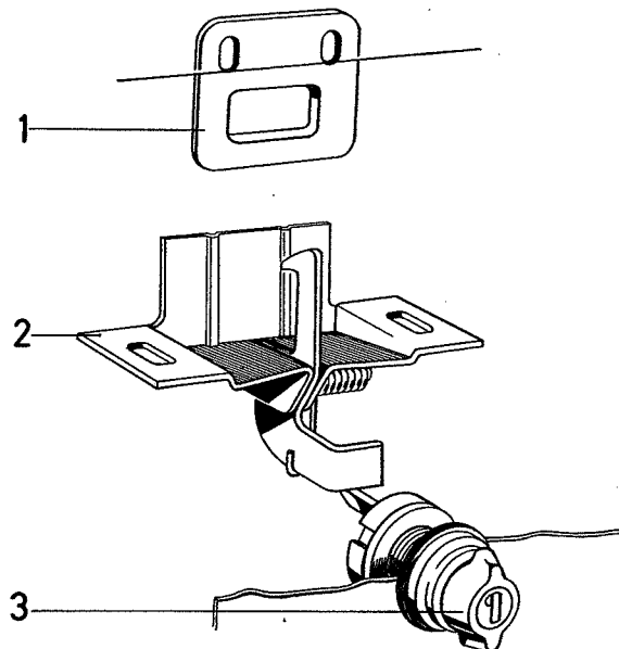
Fig. 8-15. Slot van kofferdeksel
