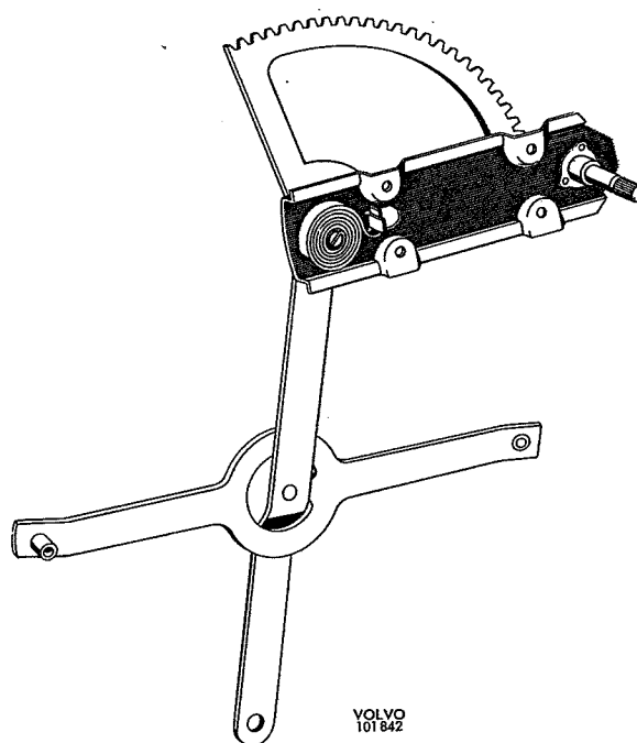
Fig. 8-13. Opdraaimechaniek
