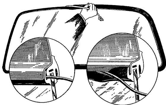
Fig. 8-23. Montage van de voorruit
