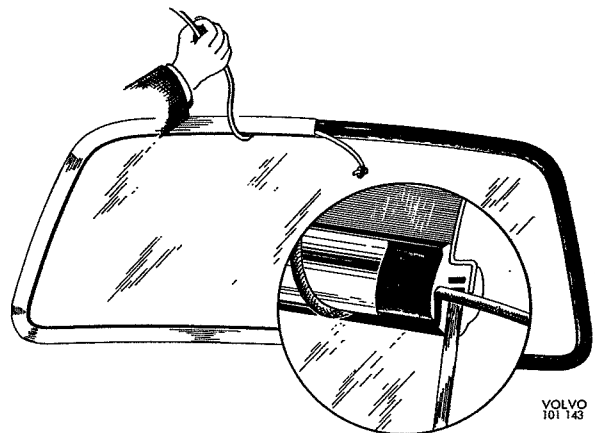
Fig. 8-18. Montage van de sierlijst
