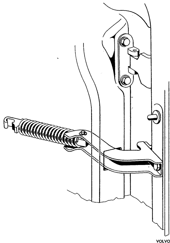
Fig. 8-5. Portierstop
