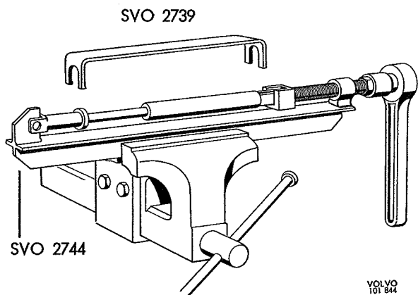
Fig. 8-14. Gereedschappen voor gascylinder
