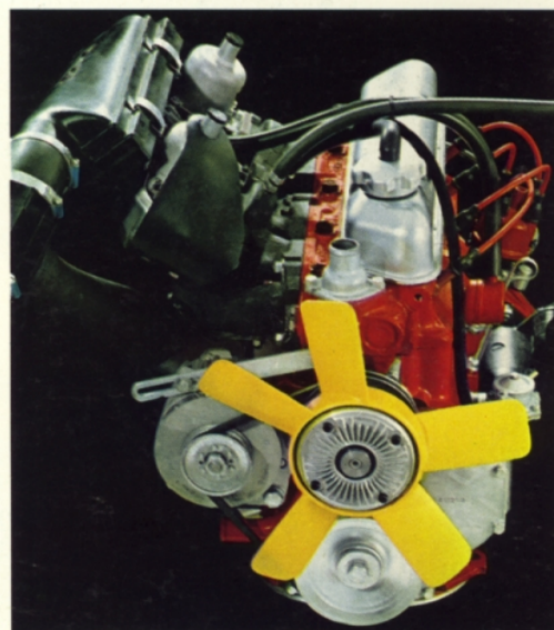
B 20 B. 2 liters, 4-cylindrig. 118 hk SAE. Avgasrening som standard. (Bilden visar motorn i utförande för Volvo 140-serien.)
