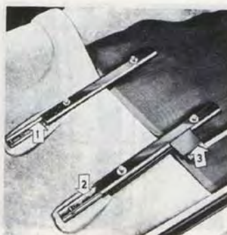
Bild 51. Stolskenor, 1800 1 och 2. Glidskenor (paraffin) 3. Spärranordning (tunn olja)
