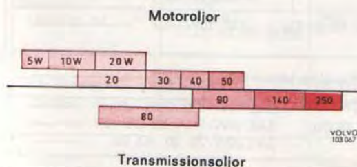
Bild 6. Viskositetsområden
