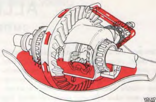
Bild 4. Oljecirkulation, bakväxel
