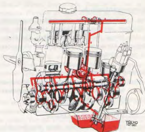
Bild 2. Smörjsystem, motor
