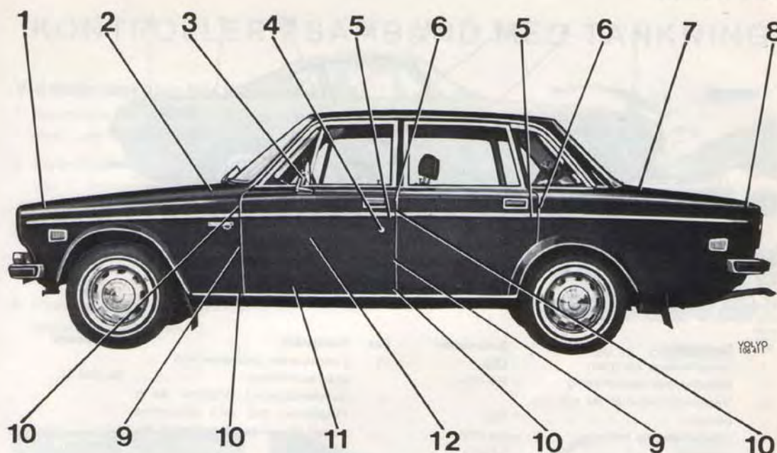
Bild 49. Smörjställen karosseri, 164
