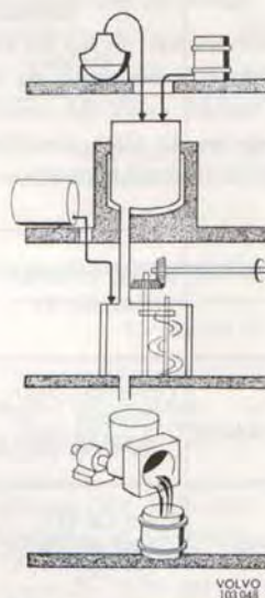
Bild 8. Princip för fettframställning
