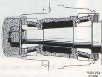
Bild 43. Framhjulslager
