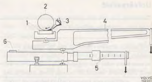
Bild 11. Princip för Timkens testmaskin
