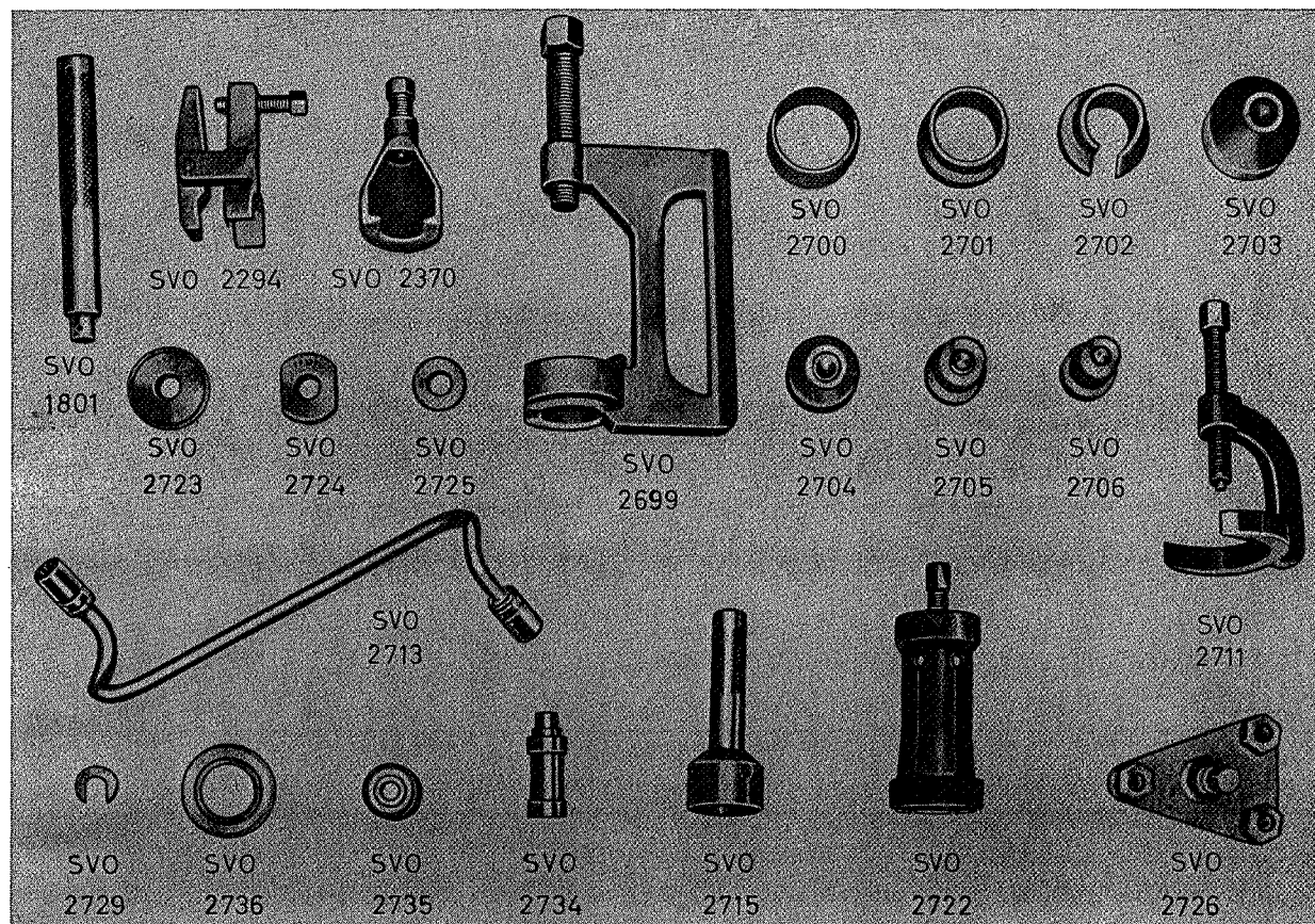
Fig. 6-1. Gereedschap voor reparatiewerkzaamheden aan de vooras
