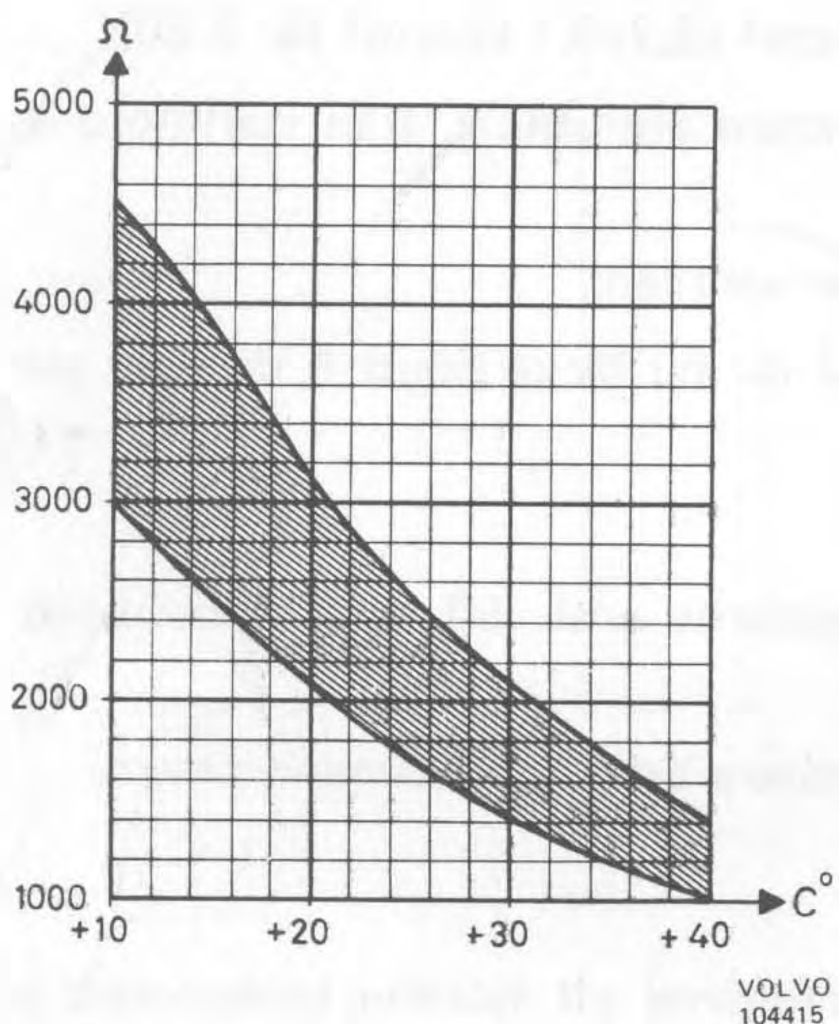
Resistans i temperaturgivare för kylvätska
