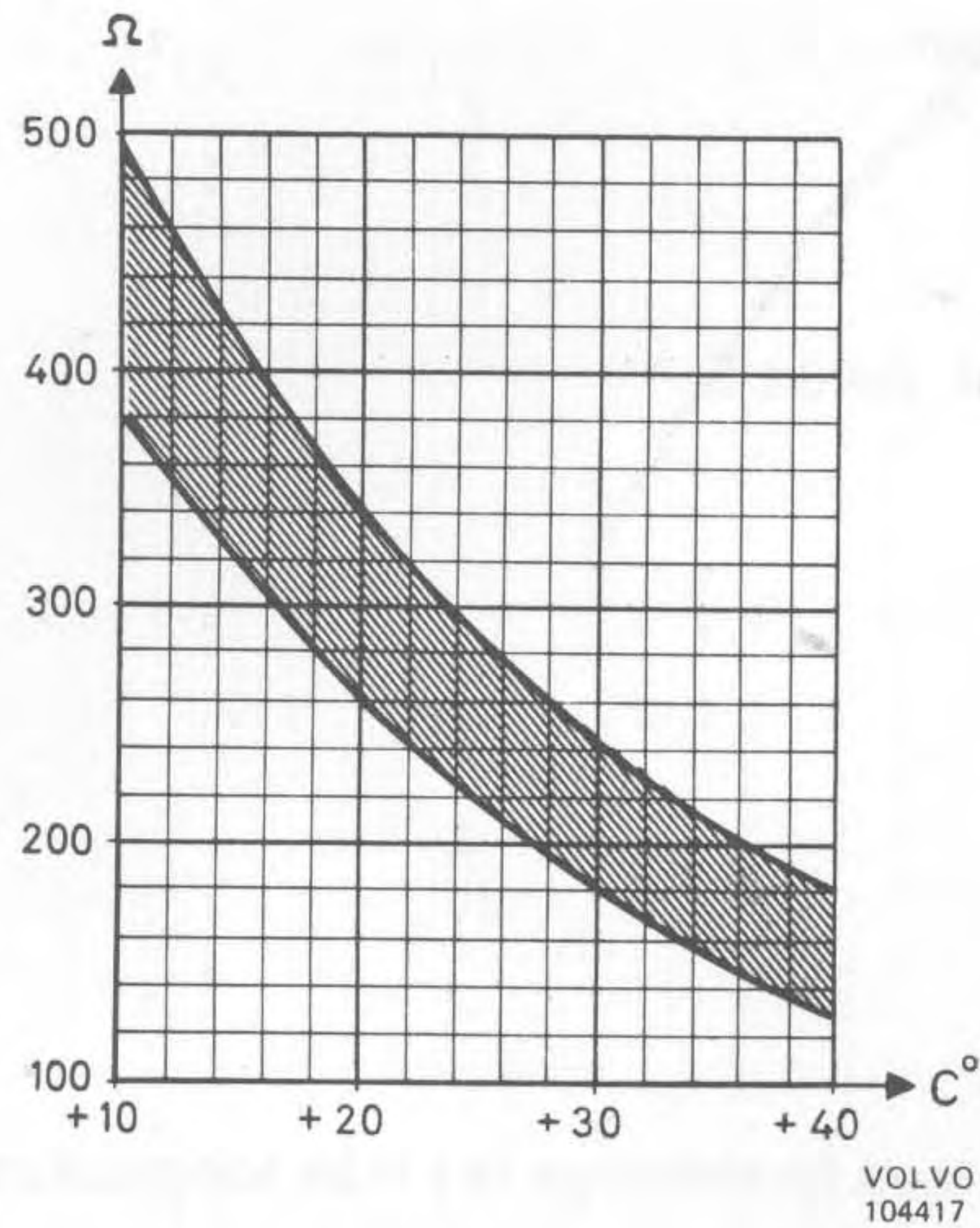
Resistans i temperaturgivare för insugningsluft
