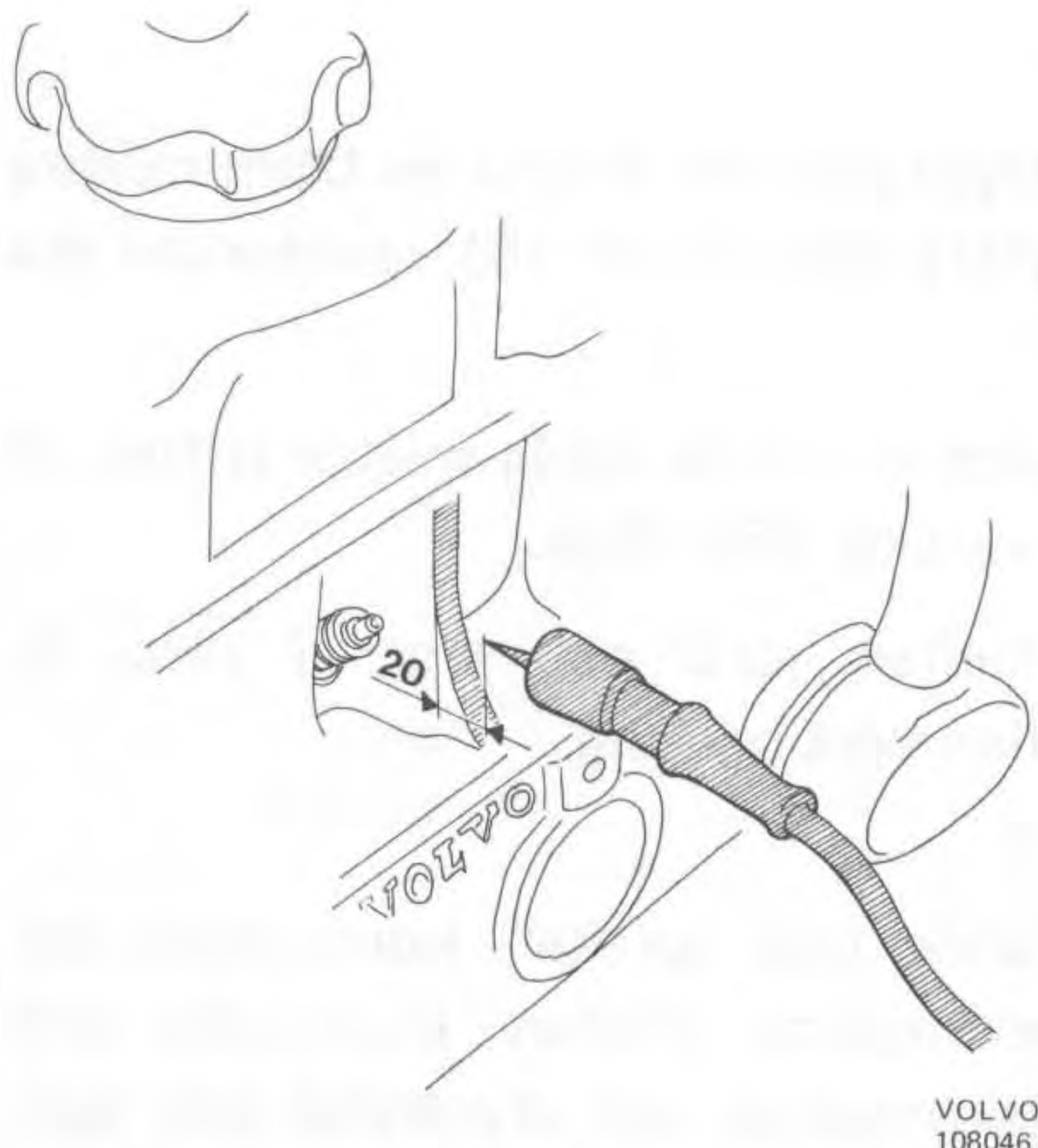
Kontroll av tändspänning utan instrument
