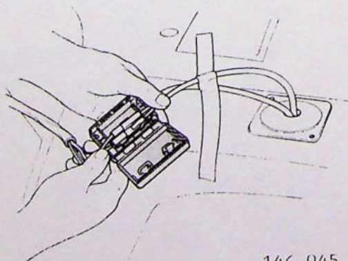
146 045 Stekerverbinding 240, 4-deurs
