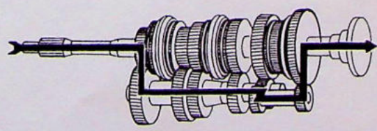
Afb. 17. Achterruit, M 51
