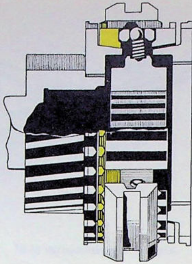
Afb. 4. Synchronisator
