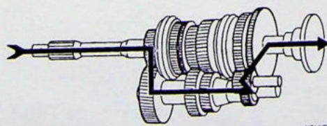
Afb. 11. Achterruit, M 50
