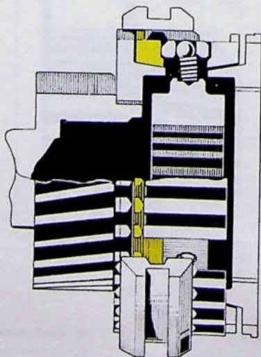
Afb. 5. Versnelling ingeschakeld
