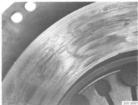
Afbeelding 1 Volledig bruikbaar
