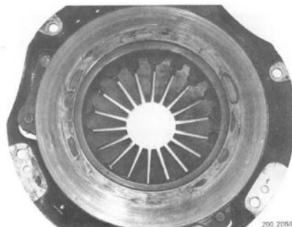
Afbeelding 8 Radiale scheurtjes
