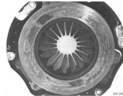
Afbeelding 4 Volledig bruikbaar
