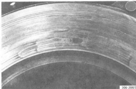
Afbeelding 7 Radiale scheurtjes
