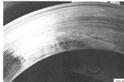
Afbeelding 5. Radiale scheurtjes
