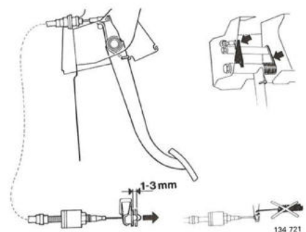
Tegenhouder Afstelmoer
