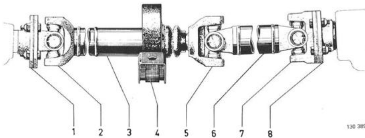
Aandrijf-as
