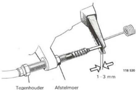
Tegenhouder Afstelmoer
