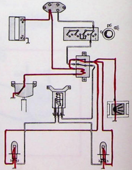
Grootlichtsignaal
