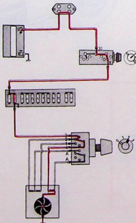
Snelheid 2
