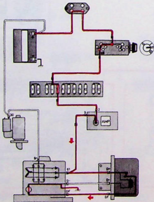
Ontsteking ingeschakeld (motor loopt niet)
