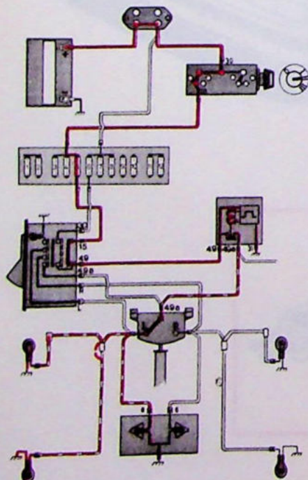
Linker richtingaanwijzer ingeschakeld
