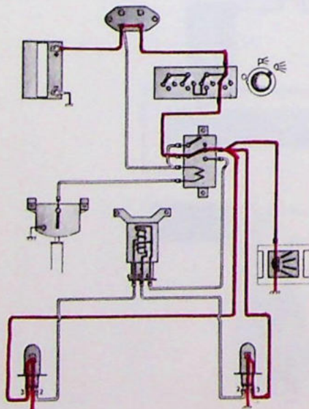
Groot licht
