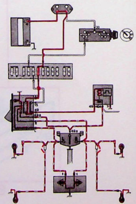
Waarschuwings- knipperlichten ingeschakeld
