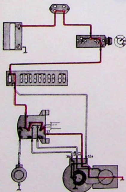
Snelheid 1
