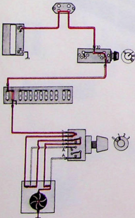
Snelheid 1
