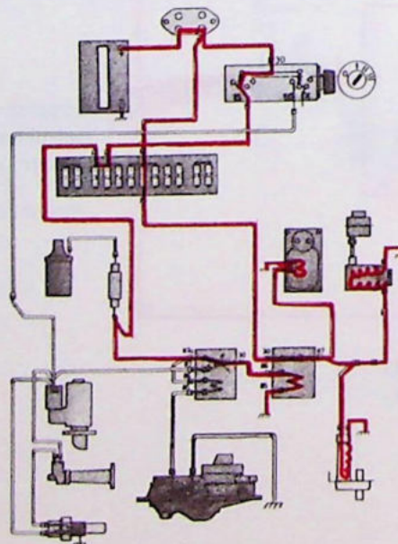
Motor loopt
