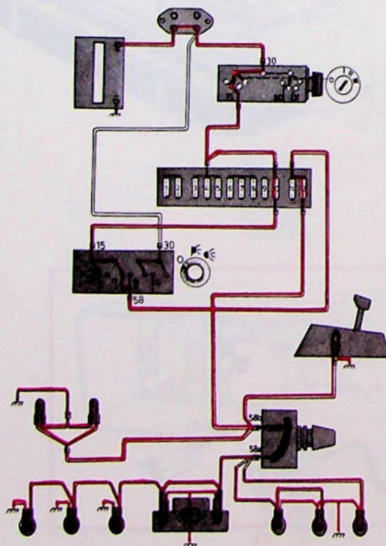
Het contact ingeschakeld
