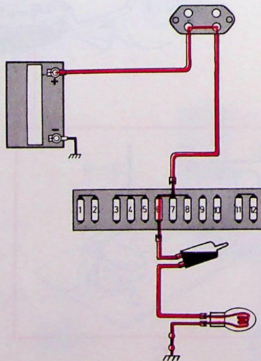
Verlichting motorruimte brandt
