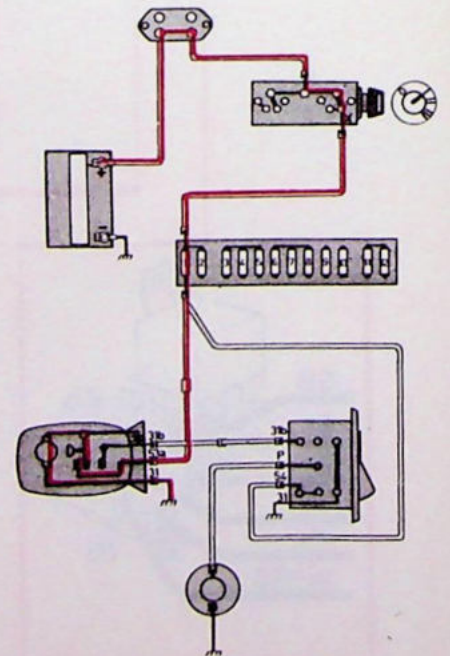
Wisser ingeschakeld (Slag na ruststand)
