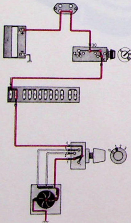
Snelheid 1
