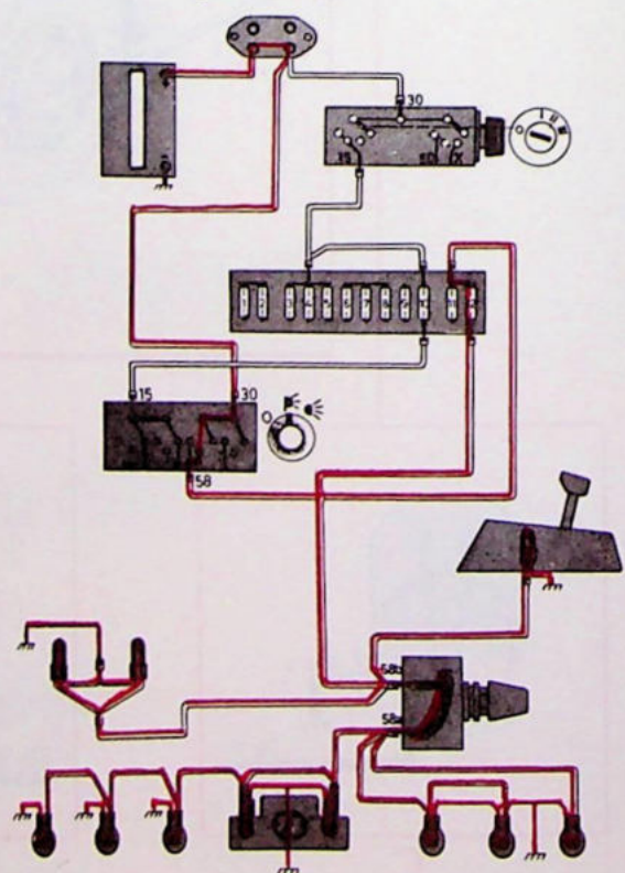
Lichtschakelaar ingeschakeld
