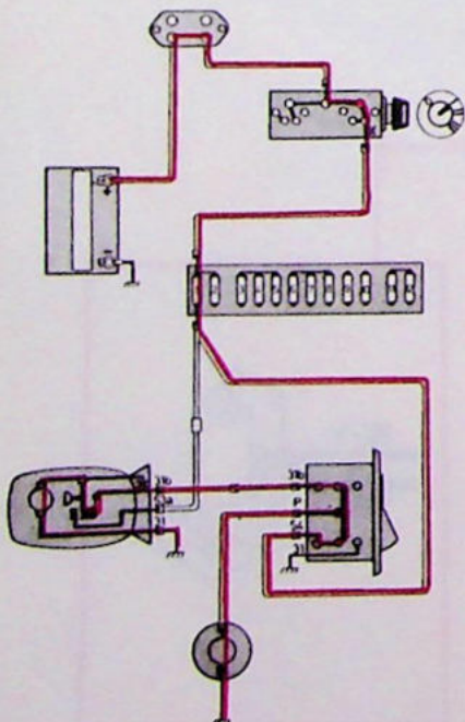
Wisser en sproeier ingeschakeld
