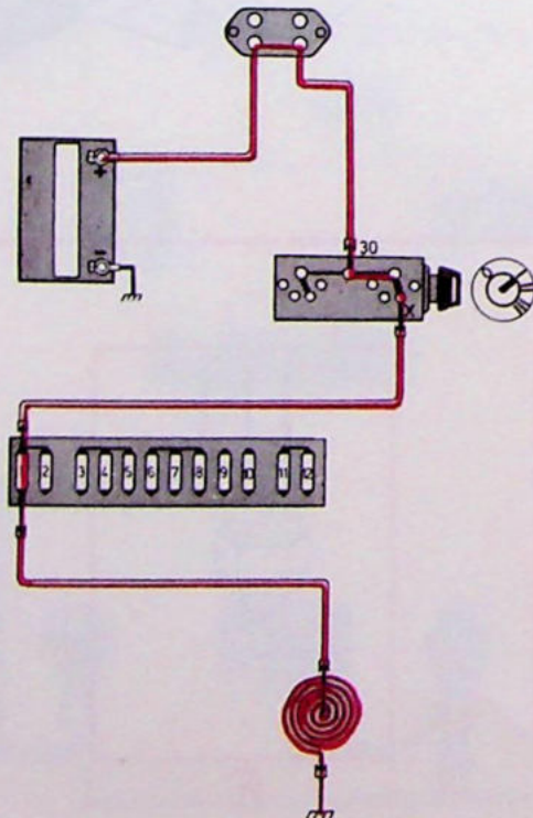
Sigaretteaansteker ingeschakeld
