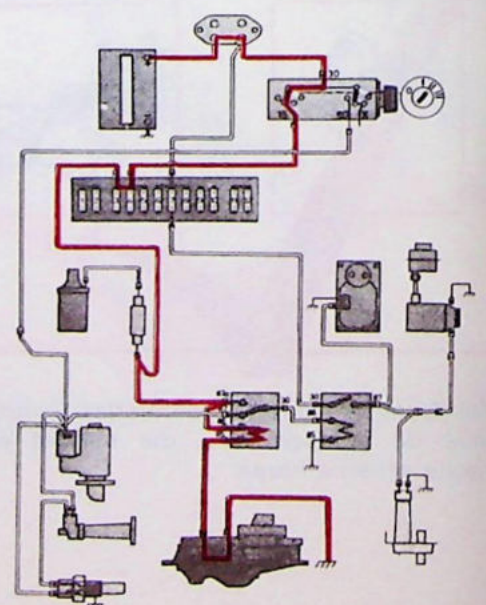
Motor afgeslagen (ontsteking ingeschakeld, maar motor loopt niet)
