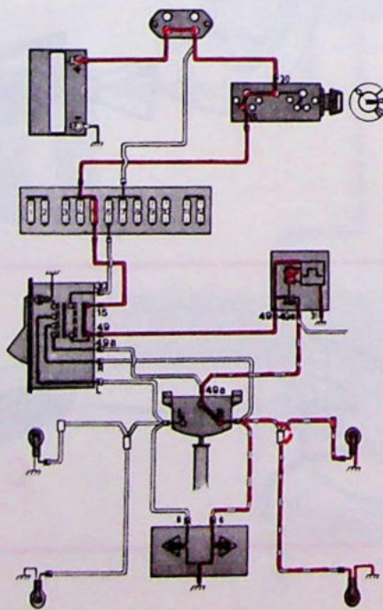
Rechter richtingaanwijzer ingeschakeld
