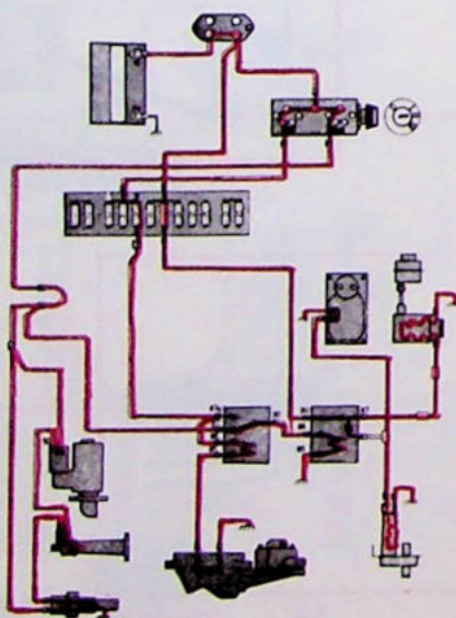
Starten van de motor
