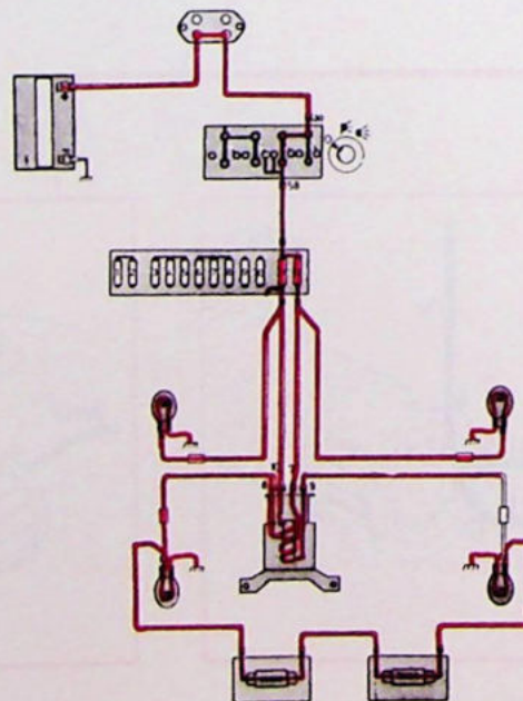
Stads- en kentekenplaatverlichting ingeschakeld
