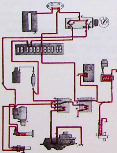
Starten van de motor
