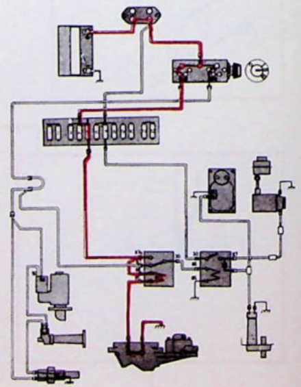
Motor afgeslagen (ontsteking ingeschakeld, maar motor loopt niet)
