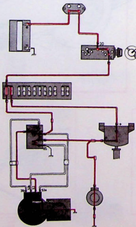
Wissers en sproeiers ingeschakeld
