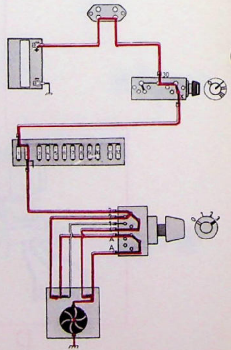
Snelheid 3
