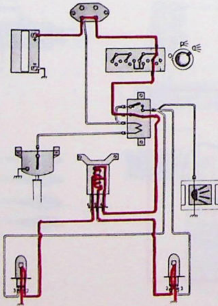
Dimlicht
