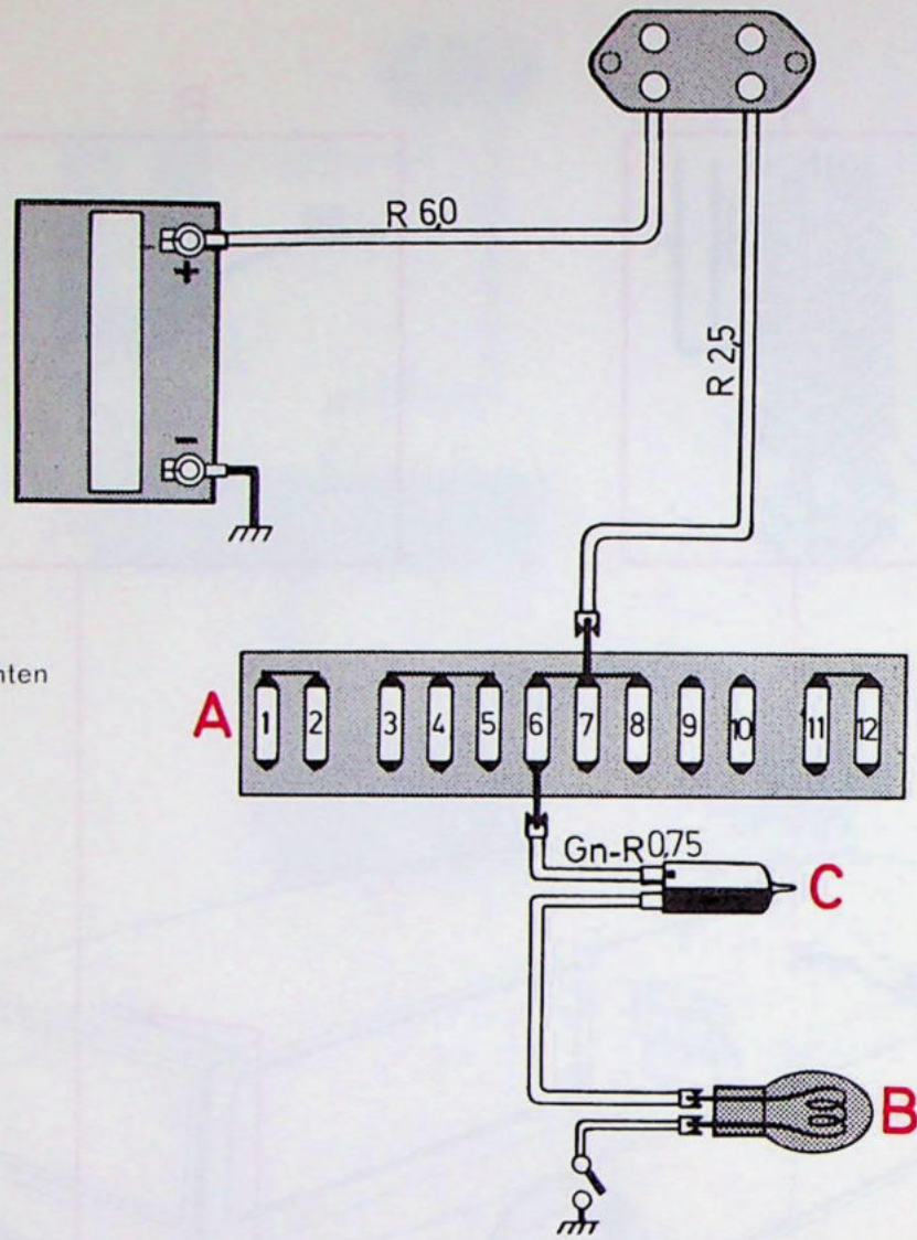
Verlichting motorruimte brandt
