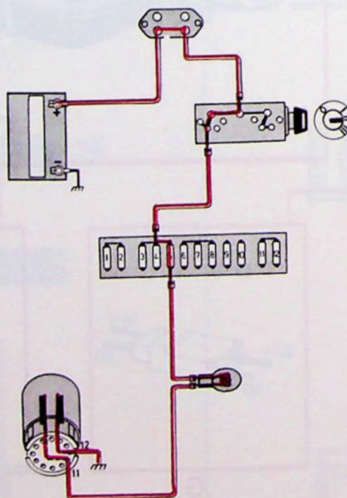
Relais ingeschakeld (één van de gloeilampen is defect)
