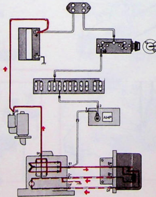
Dynamo laadt
