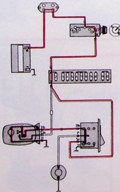
Wisser ingeschakeld
