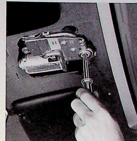
Druk het plastic pannetje in en draai.
