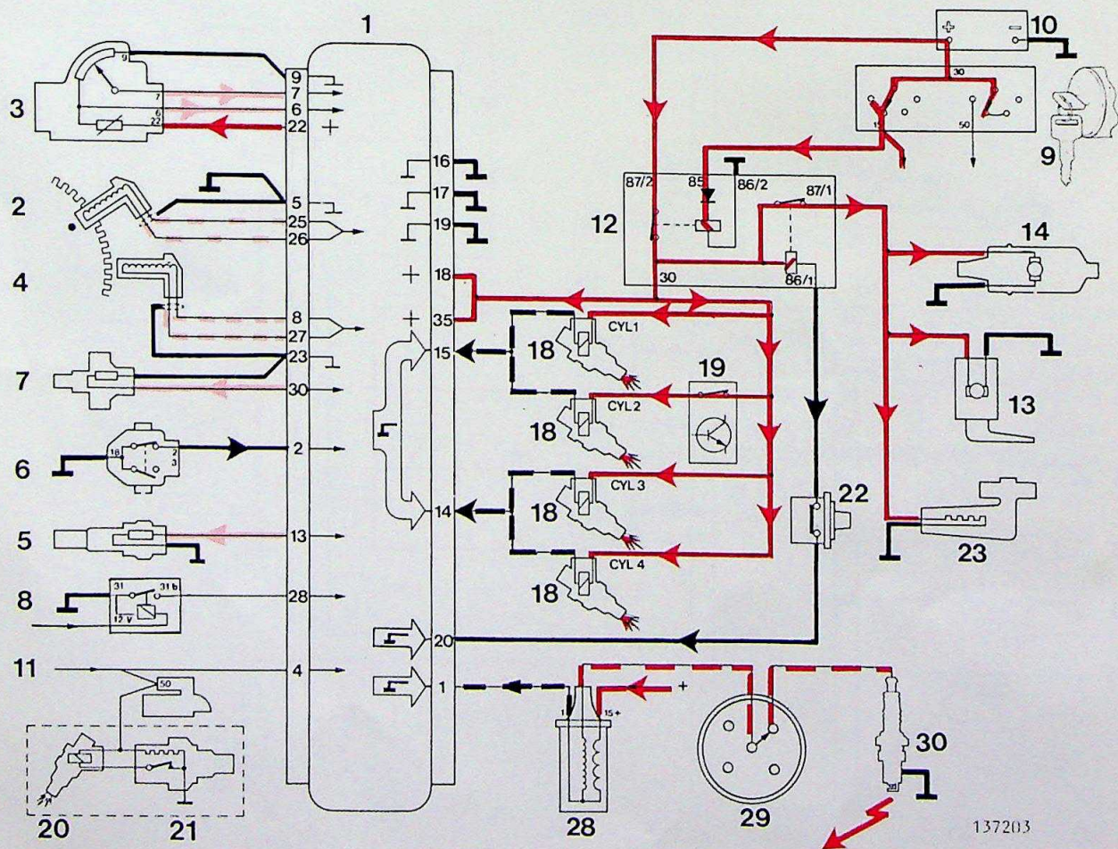
Principetekening, zonder aansluitstukken en zekeringen
