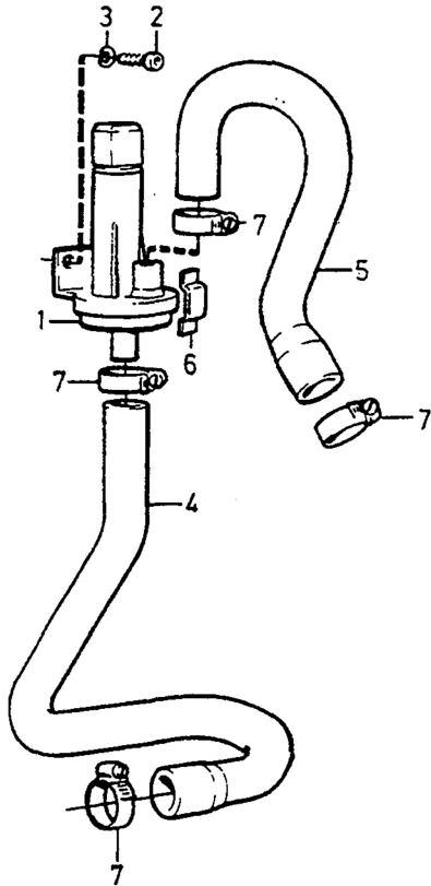
4 CYL ALTER 1
