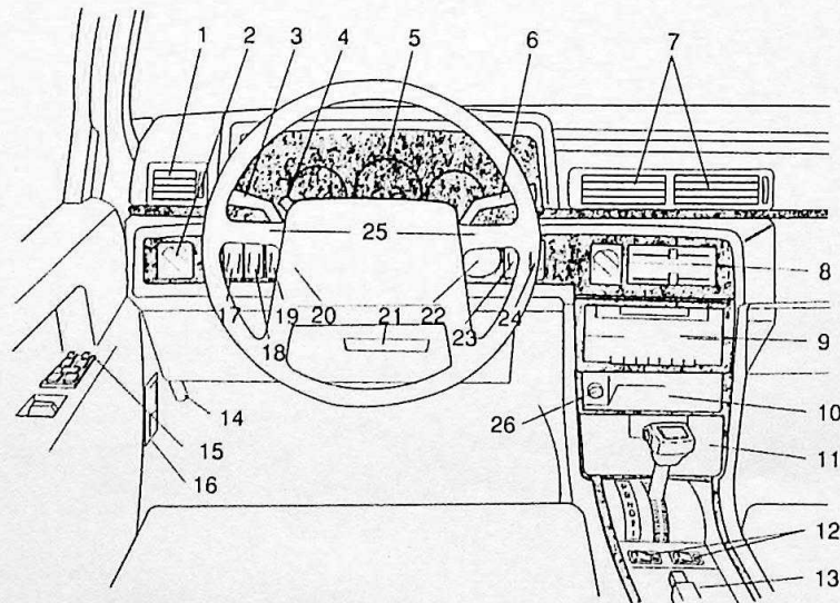
Figuur 1.5: Dashboard van de Volvo 740
