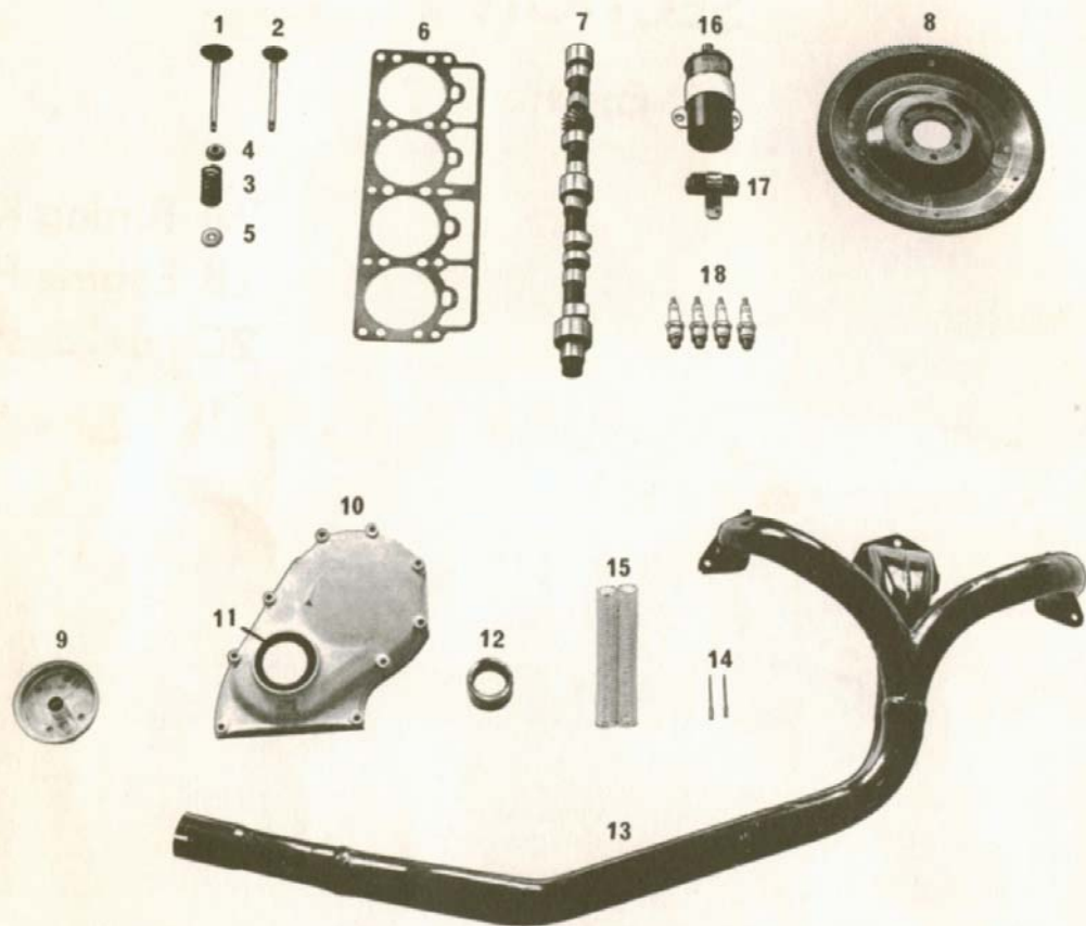
Trimmingsdetaljer för motor B18
