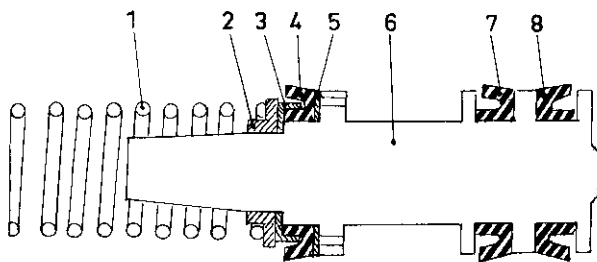
Abb. 57 Sekundärkolben
