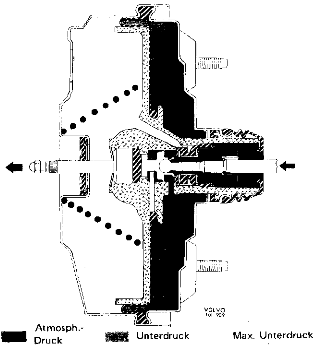
Abb. 84 Teilbremsstellung
