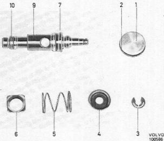
Abb. 90 Teile des Regulierkolbens
