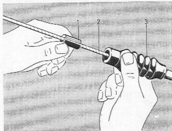
Abb. 111 Aufziehen der Gummimanschette
