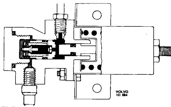
Abb. 47 Druckreduzierung
