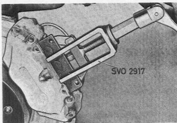
Abb. 18 Ausbau des Bremsklötzes
