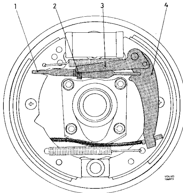
Abb. 16 Selbsttätige Nachstellvorrichtung
