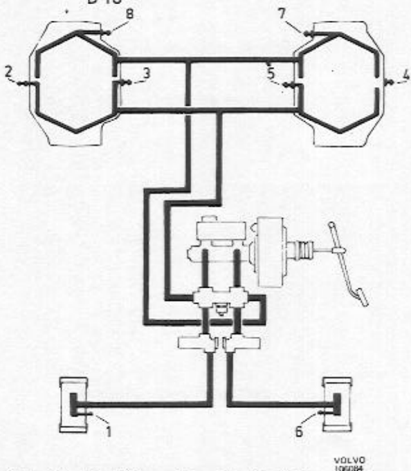
Abb. 70 Entlüftungsfolge, Zweikreis-Bremsanlage, B 20
