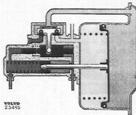
Abb. 80 Dauerbremsung
