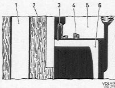
Abb. 11 Ruhelage
