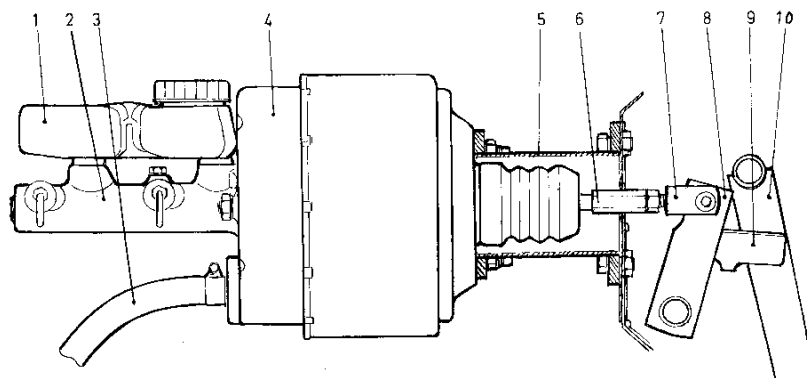
Abb. 105 Bremsteile, 1800
