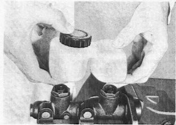
Abb. 51 Ausbau des Tandembehälters
