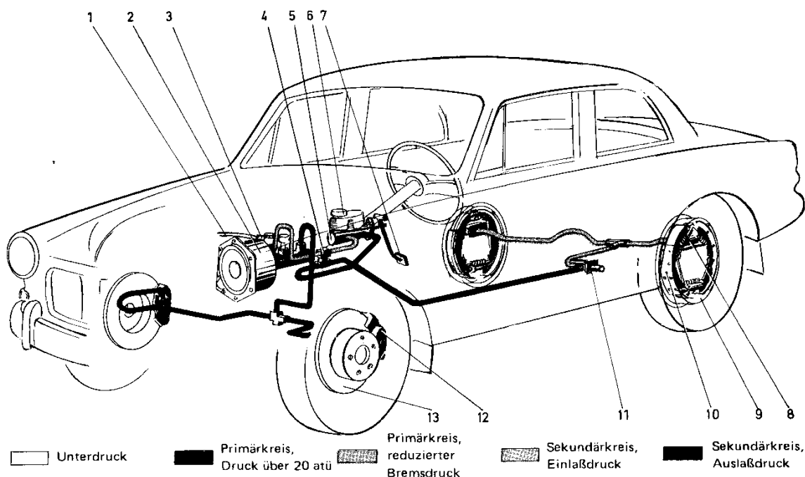
Abb. 6 Zweikreis-Fußbremsanlage, B 18
