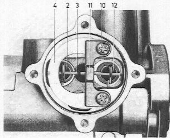
Abb. 97 Ventile eingebaut
