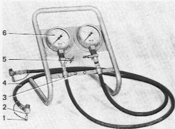
Abb. 2 Bremsdruck-Prüfgerät 999 2741
