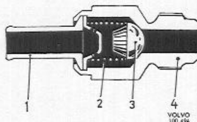
Abb. 86 Rückschlagventil
