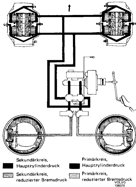
Abb. 35 Bremsse angesetzt
