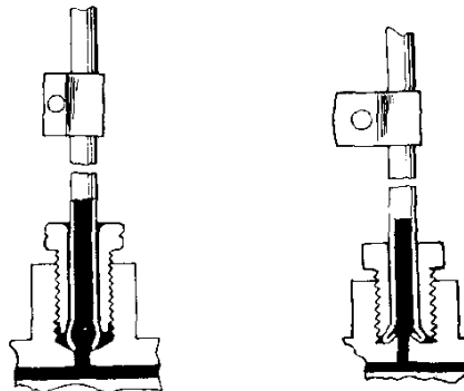
Abb. 67 Anschlußteile
