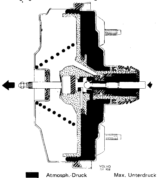
Abb. 83 Vollbremsstellung
