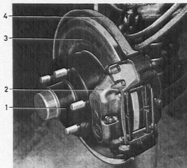
Abb. 8 Bremssteile, Vorderrad
