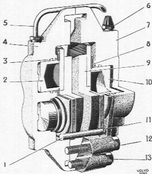
Abb. 9 Vorderer Bremssattel
