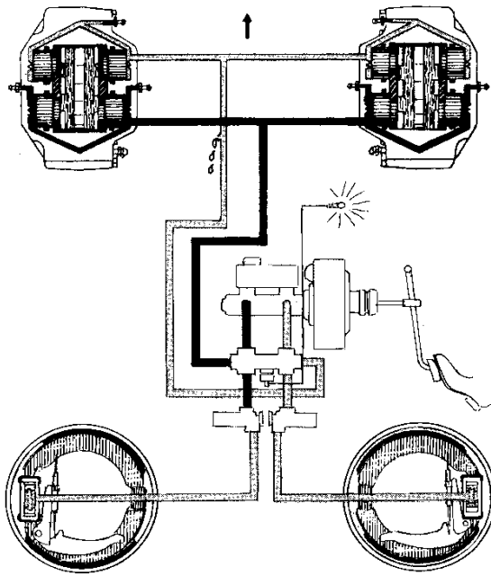
Abb. 36 Bremse angesetzt (undichter Sekundärkreis)
