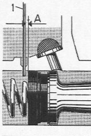
Abb. 50 Kontrolle der Ausgleichbohrung
