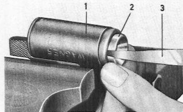
Abb. 29 Kontrolle des Kolbenspiels im Radbremszylinder
