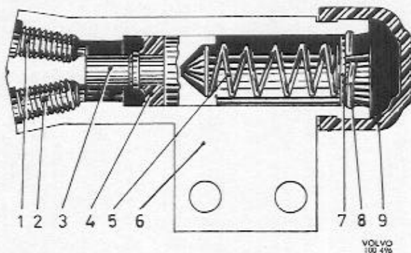
Abb. 100 Steuerzylinder
