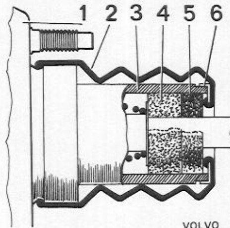
Abb. 103 Filterbestandteile
