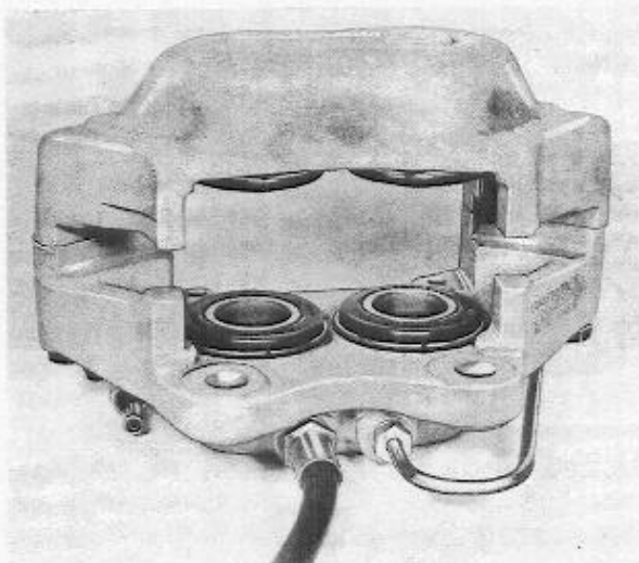
Abb. 24 Vorderer Bremsattel, zusammengebaut
