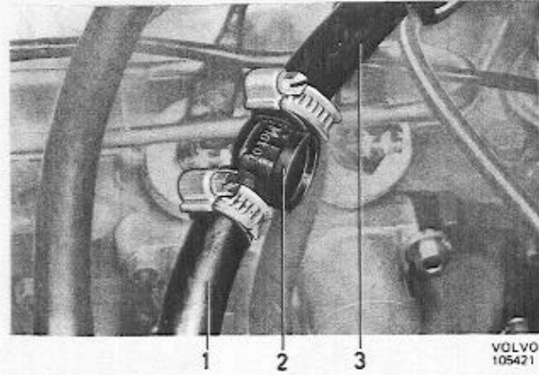
Abb. 108 Rückschlagventil, Typ 3
