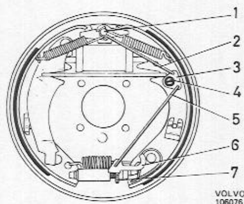
Abb. 31 Hinterradbremse, Zweikreis-Bremsanlage, B 18
