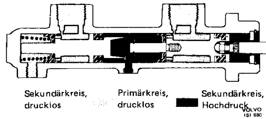
Abb. 40 Bremsansetzung (undichter Sekundärkreis)
