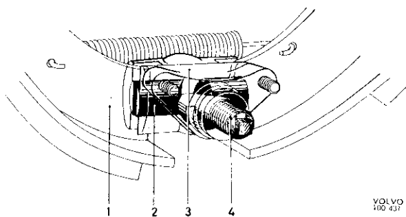
Abb. 14 Einstellvorrichtung
