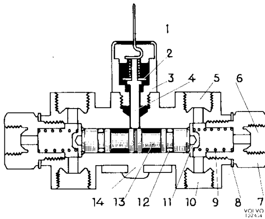
Abb. 42 Warnventil
