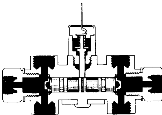
Abb. 43 Normalstellung
