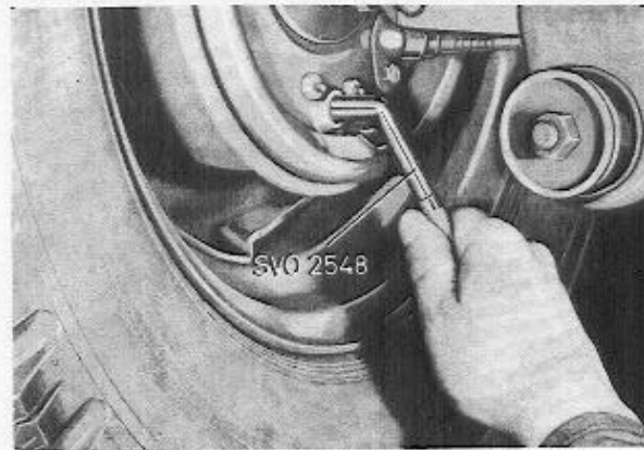
Abb. 32 Einstellung der Hinterradbremse
