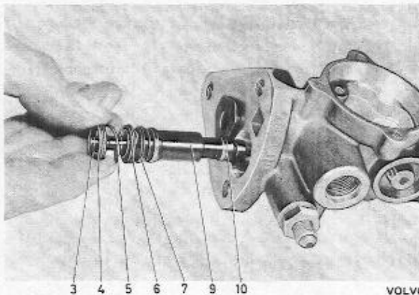
Abb. 96 Einbau des Regulierkolbens
