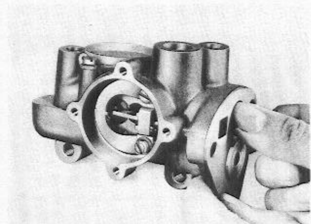
Abb. 98 Prüfung des Reguliermechanismus
