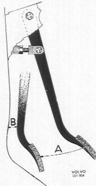
Abb. 73 Hub des Bremspedals
