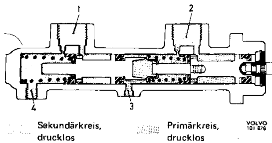
Abb. 38 Ruhelage
