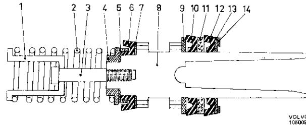
Abb. 58 Primärkolben
