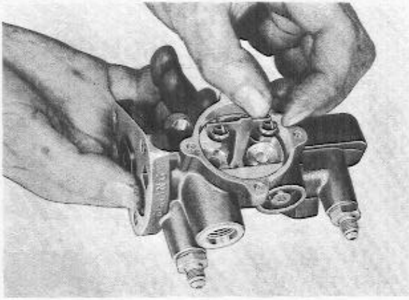
Abb. 89 Ausbau des Ventilhebels
