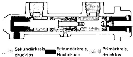
Abb. 41 Bremsansetzung (undichter Primärkreis)
