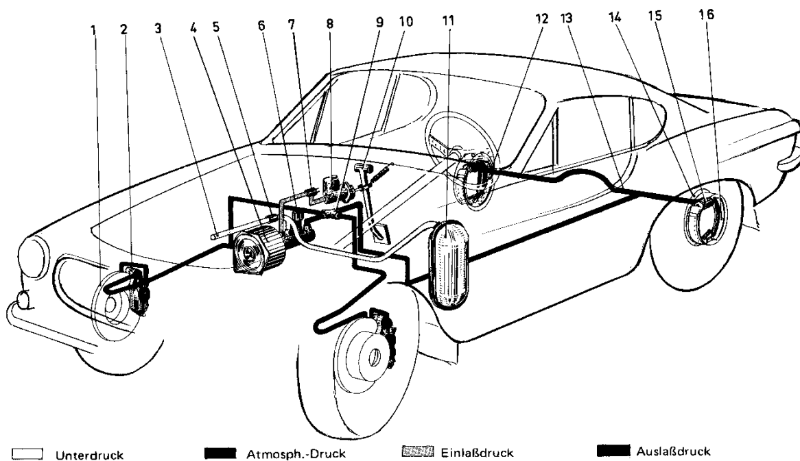
Abb. 5 Einkreis-Fußbremsanlage
