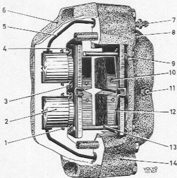
Abb. 10 Bremssattel für Zweikreis-Bremsanlage, B 20
