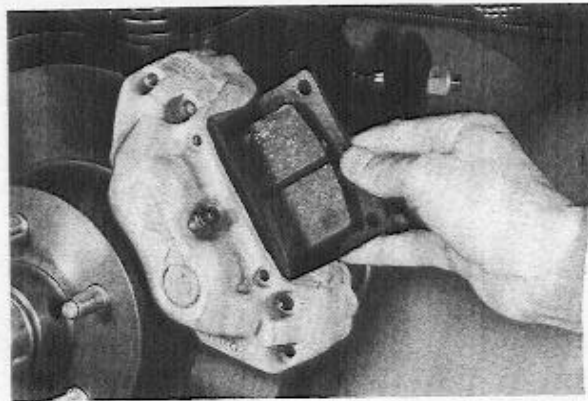
Abb. 19 Einbau des Bremsklötzes
