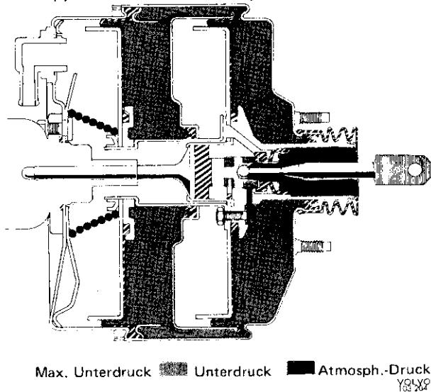
Abb. 85 Servobremsszylinder, Typ 2
