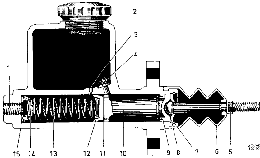
Abb. 37 Hauptzylinder, Einkreis-Bremsanlage
