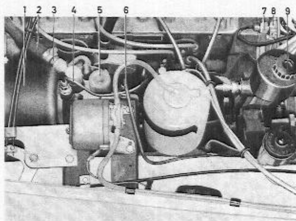
Abb. 88 Bremssteile im Motorraum, P 1800 (ab Fahrgestell-Nr. 7000)
