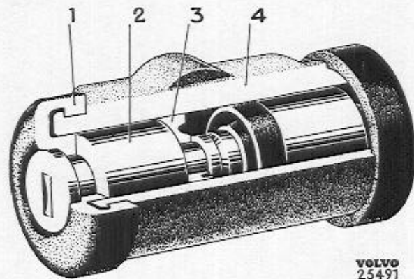
Abb. 13 Radbremszylinder, Hinterrad
