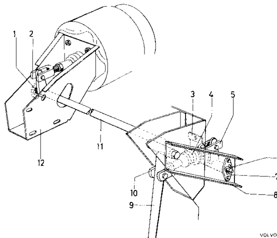
Abb. 106 Bremsteile, rechtsgelenkte Ausführung
