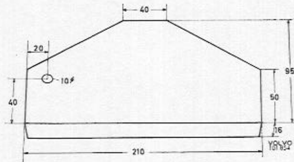
Abb. 3 Holzscheibe für Bremssattel
