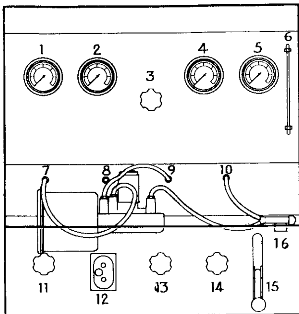
Abb. 99 Prüfstandanschlüsse
