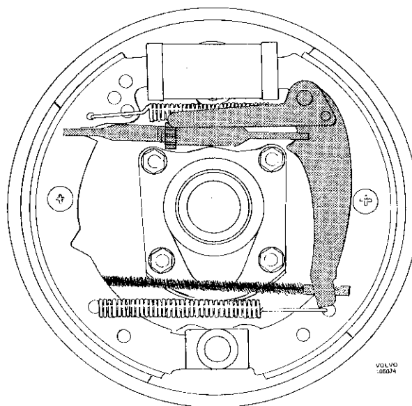
Abb. 17 Bremsansetzung
