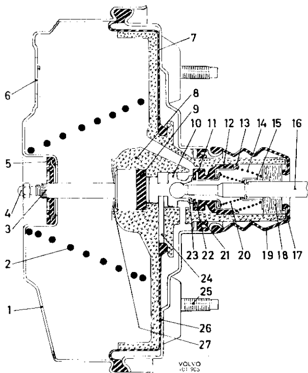
Abb. 81 Servobremsszylinder, Typ 2
