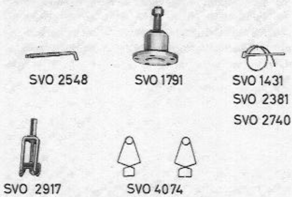
Abb. 1 Spezialwerkzeug
