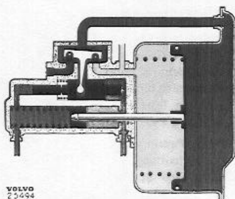
Abb. 79 Bremsansetzung
