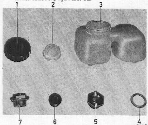
Abb. 52 Teile zum Behälter
