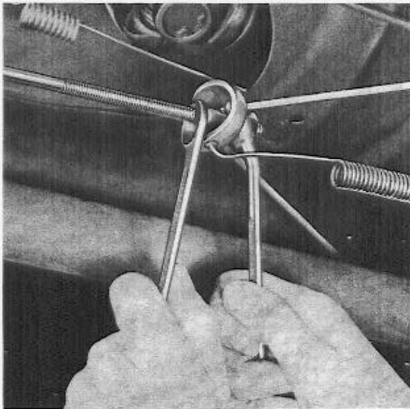
Abb. 110 Einstellen der Handbremse
