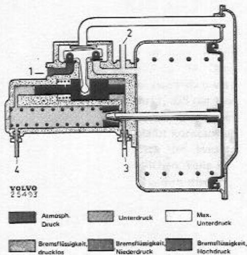
Abb. 78 Ruhestellung
