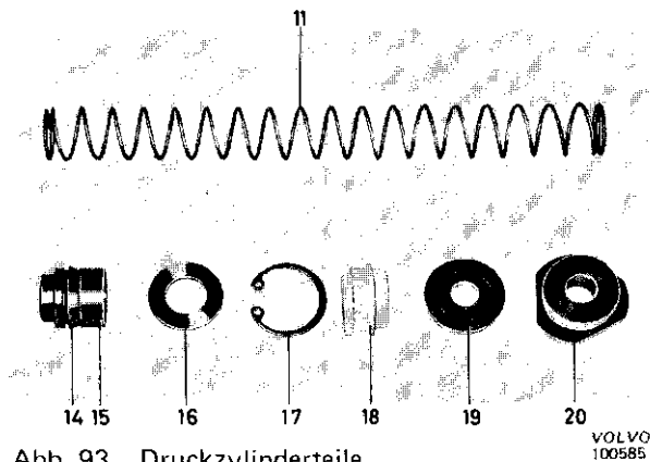
Abb. 93 Druckzylinderteile
