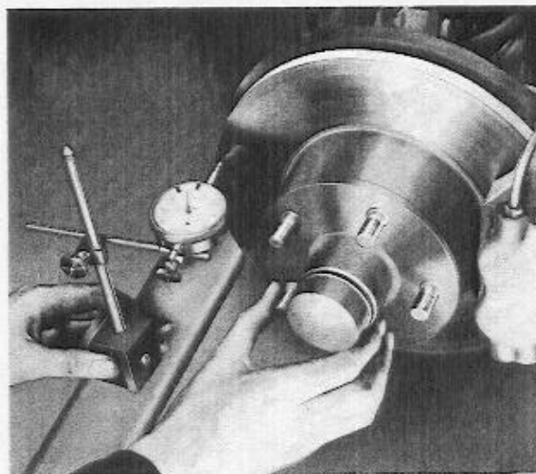
Abb. 25 Kontrollmessung des Seitenschlages
