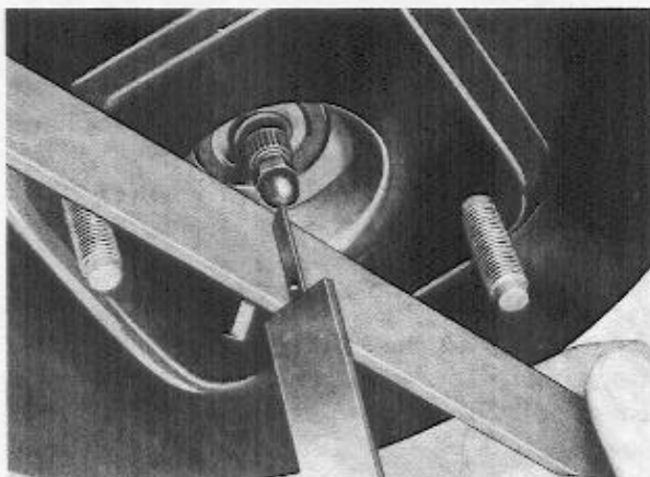
Abb. 60 Messen der Druckstange (Höhe über Flanschebene)
