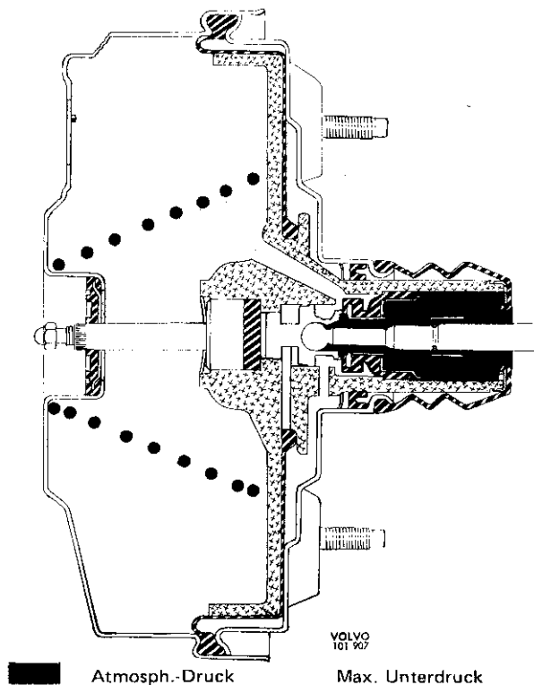
Abb. 82 Ruhestellung
