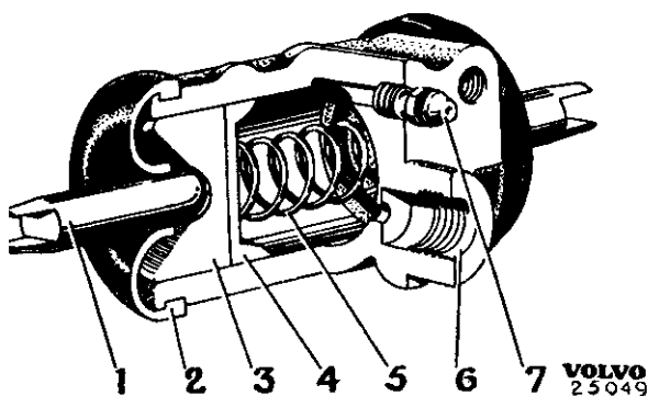
Abb. 15 Radbremszylinder, Typ Duo-servo
