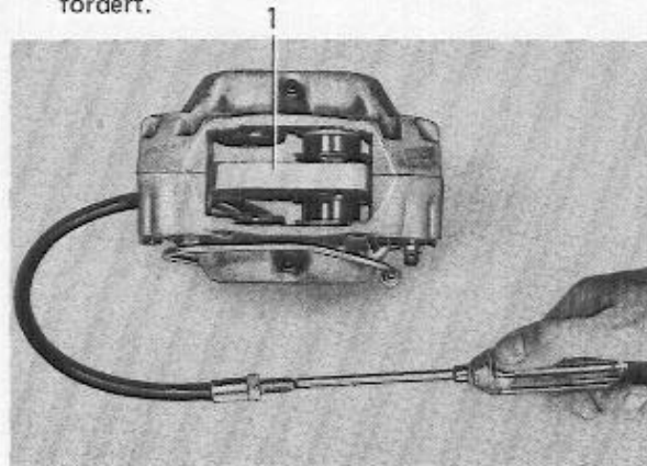
Abb. 22 Ausbau der Kolben
