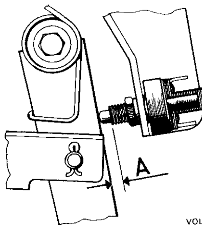
Abb. 76 Einstellung des Bremslichtschalters A = 2–6 mm
