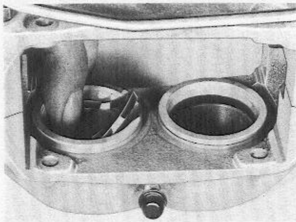
Abb. 23 Einbau des Dichtringes
