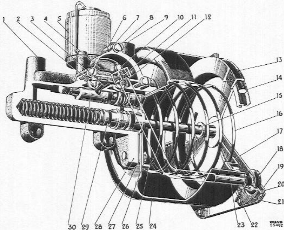
Abb. 77 Servobremsszylinder, Typ 1
