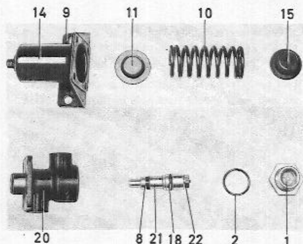
Abb. 65 Bremskraftregler, zerlegt
