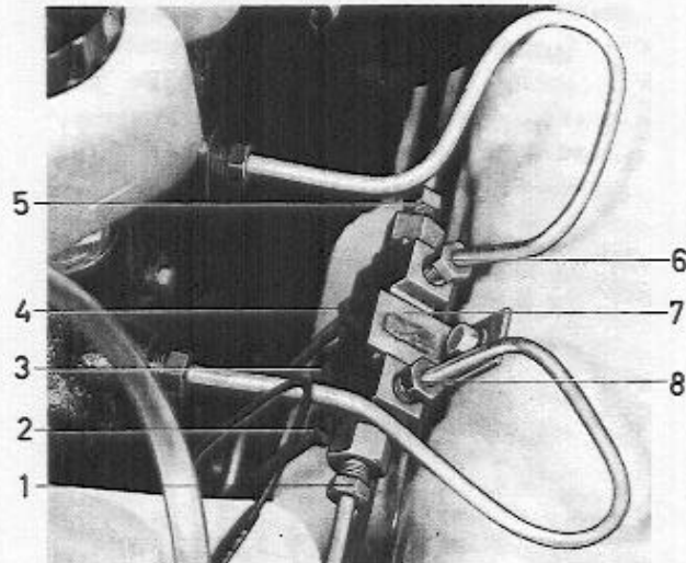
Abb. 62 Warnventil eingebaut
