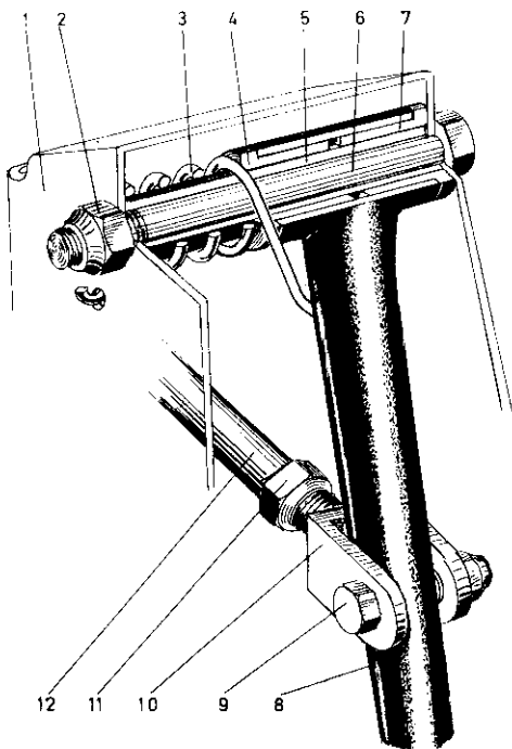
Abb. 74 Pedallagerung, 120
