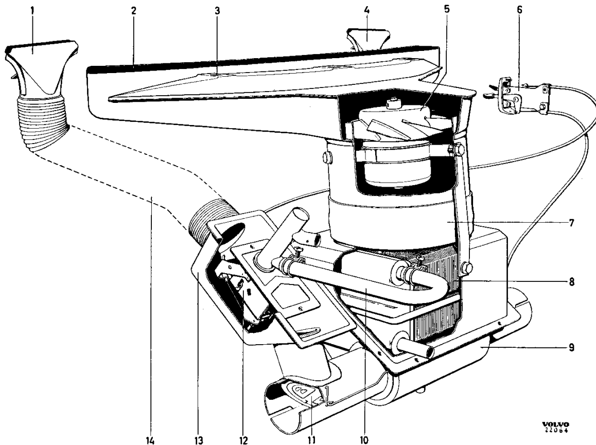
Abb. 17 Heizgebläse
