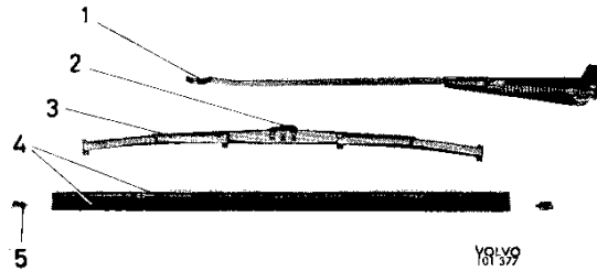
Abb. 9 Scheibenwischerarm mit komplettem Wischerblatt
