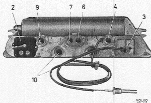
Abb. 3 Kombinationsinstrument, Hinterseite
