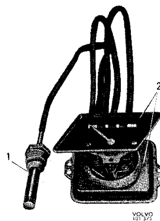
Abb. 7 Kühlwasser – Fernthermometer
