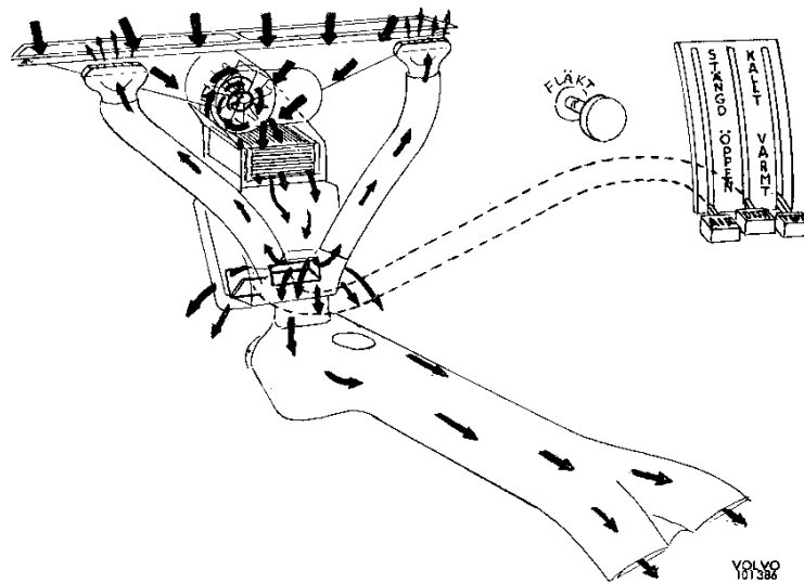
Abb. 19 Aufbau und Funktion der Heizung
