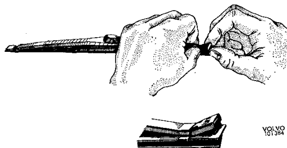
Abb. 16 Auswechseln des Wischerblattes
