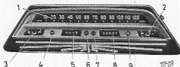
Abb. 2 Kombinationsinstrument, Vorderseite
