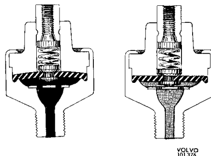
Abb. 8 Funktion des Öldruck – Wächters
