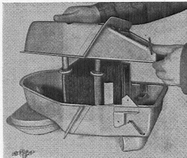
Abb. 22 Zerlegung des Heizgebläses
