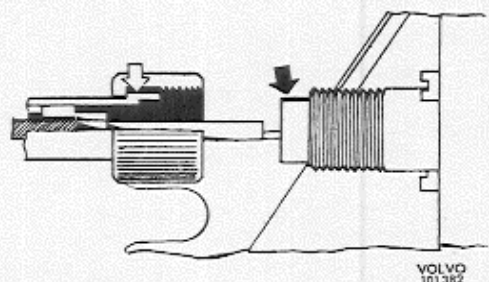
Abb. 14 Anschluß der Tachometerwelle, spätere Ausführung
