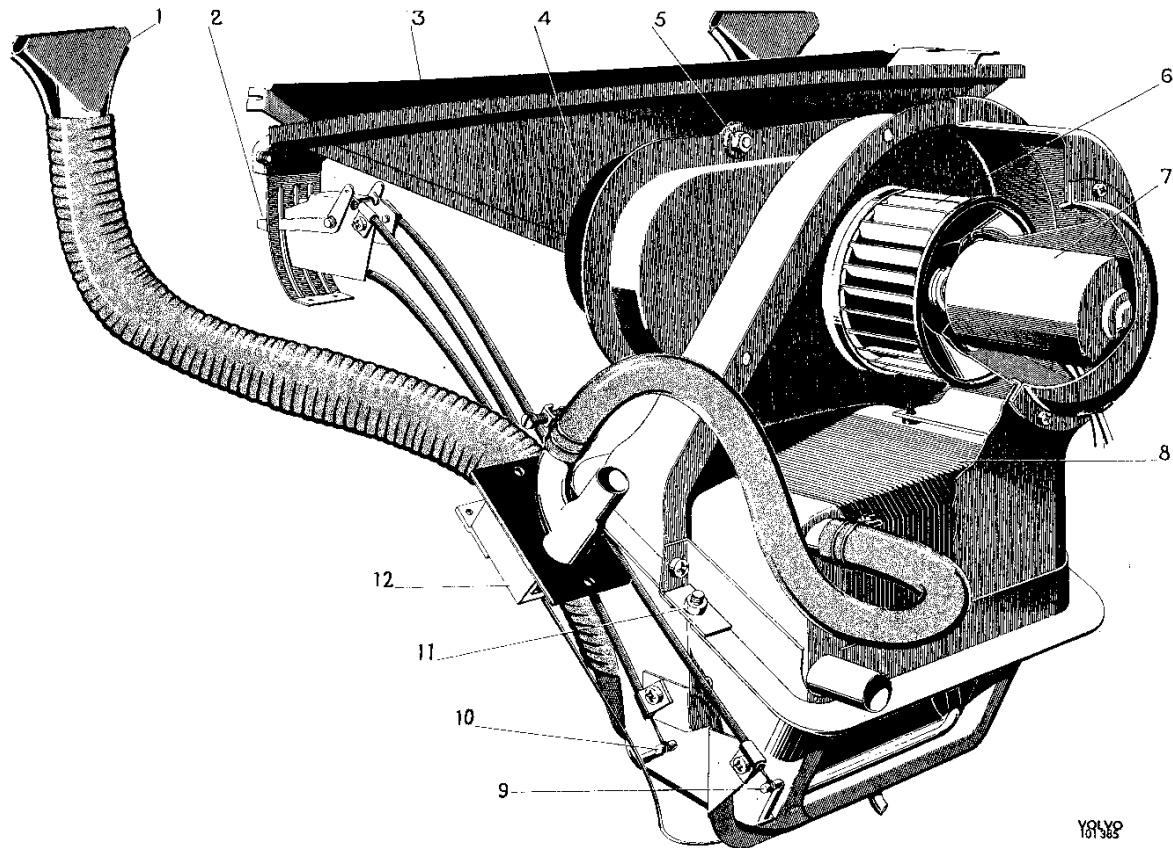
Abb. 18 Heizgebläse
