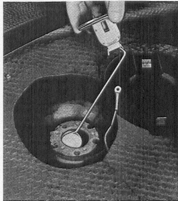
Abb. 11 Ausbau des Kraftstoffstandgebers
