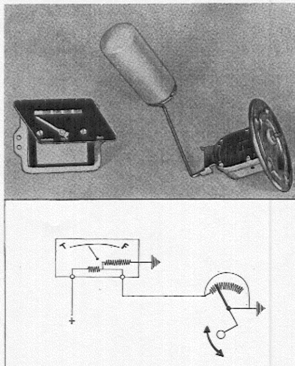
Abb. 4 Kraftstoffanzeiger
