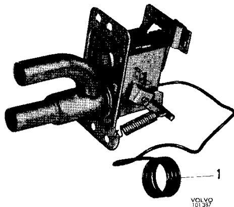
Abb. 20 Wärmekontrollventil
