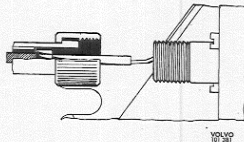
Abb. 13 Anschluß der Tachometerwelle, frühere Ausführung
