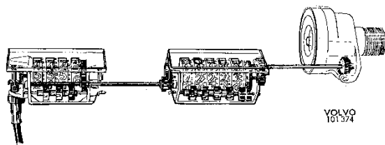
Abb. 6 Prinzipskizze, Antrieb von Kilometer-bzw. Teilstreckenzähler
