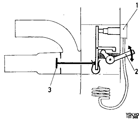
Abb. 21 Vereinfachte Skizze der Arbeitsweise des Wärmekontrollventiles
