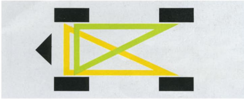
Zweikreis-Bremssystem „2 X 3“: Jeder Kreis wirkt auf beide Vorderräder und je ein Hinterrad.
