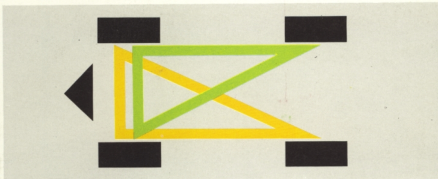
2-krets bromssystem. Triangeldelet. Skadas en krets har Ni likväl 3 bromsande hjul på den andra. Behåller ca 80 % av bromsverkan.
