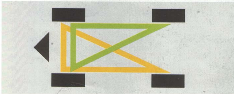
2-krets bromssystem. Triangeldelat. Skadas en krets har Ni likväl 3 bromsande hjul på den andra. Behåller ca 80 % av bromsverkan.
