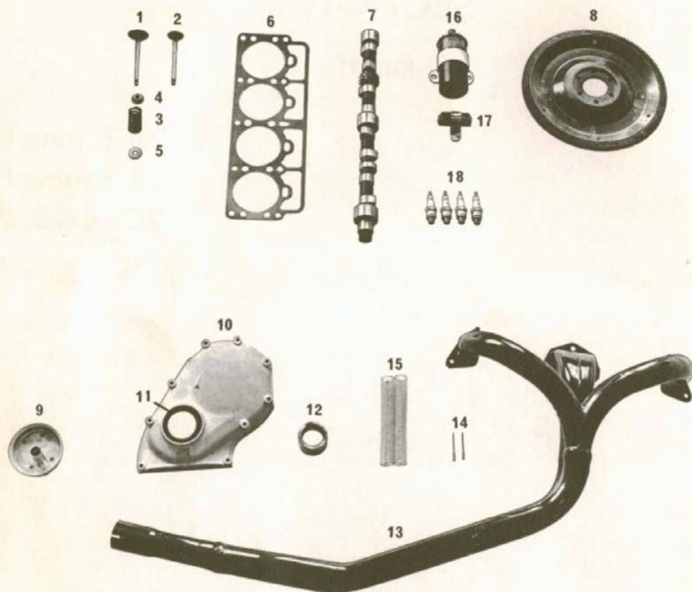
Trimningsdetaljer för motor B18
