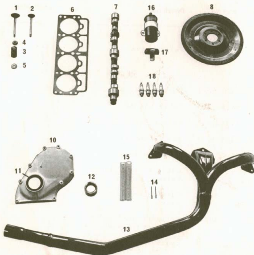
Trimningsdetaljer för motor B18
