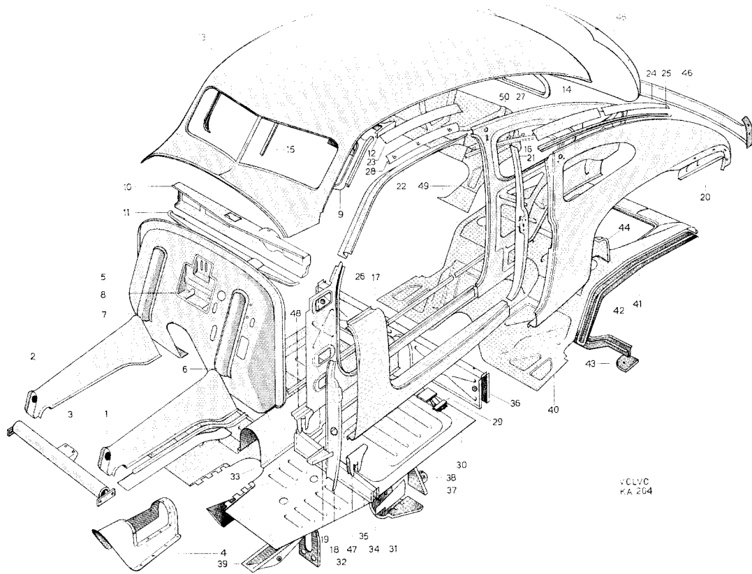
Fig. 21. Body assembly
