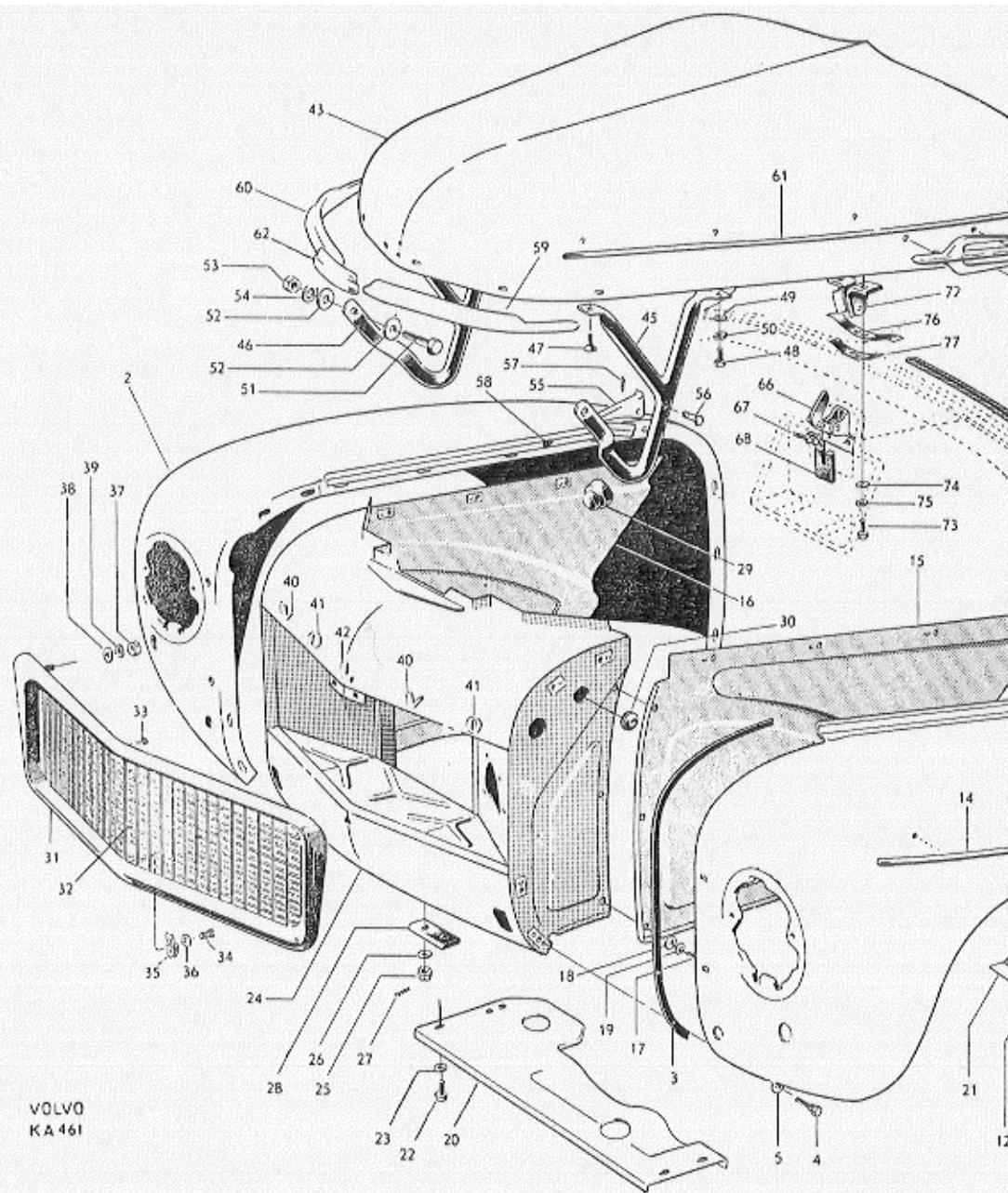
Bild nr 40 Plåtetaljer på karoseri
