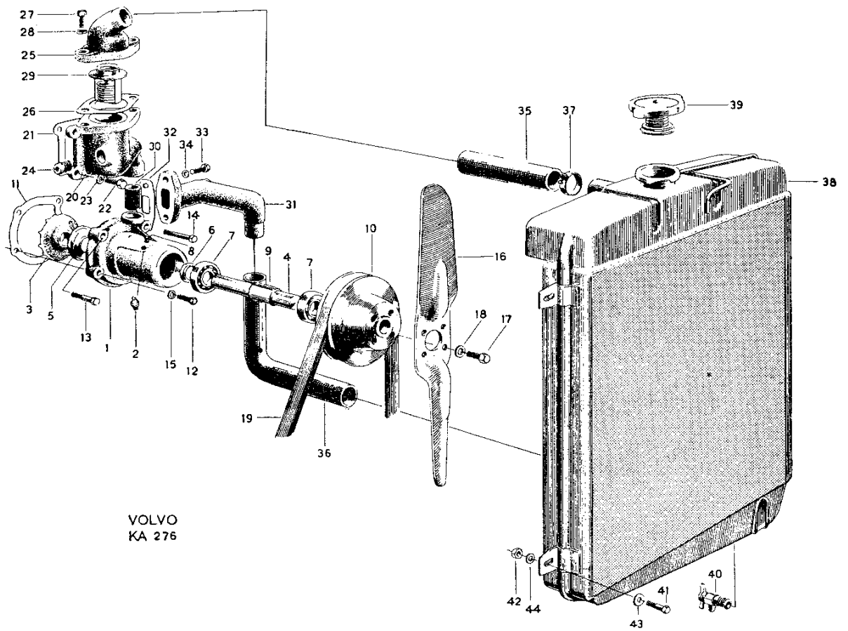
Bild nr 9 Kylsystem
