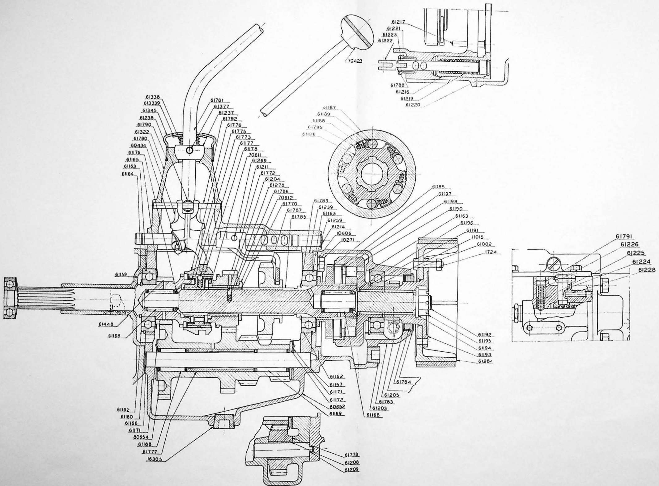
Fig. 176. Frijhjulsväxellåda, det. nr 61380.
