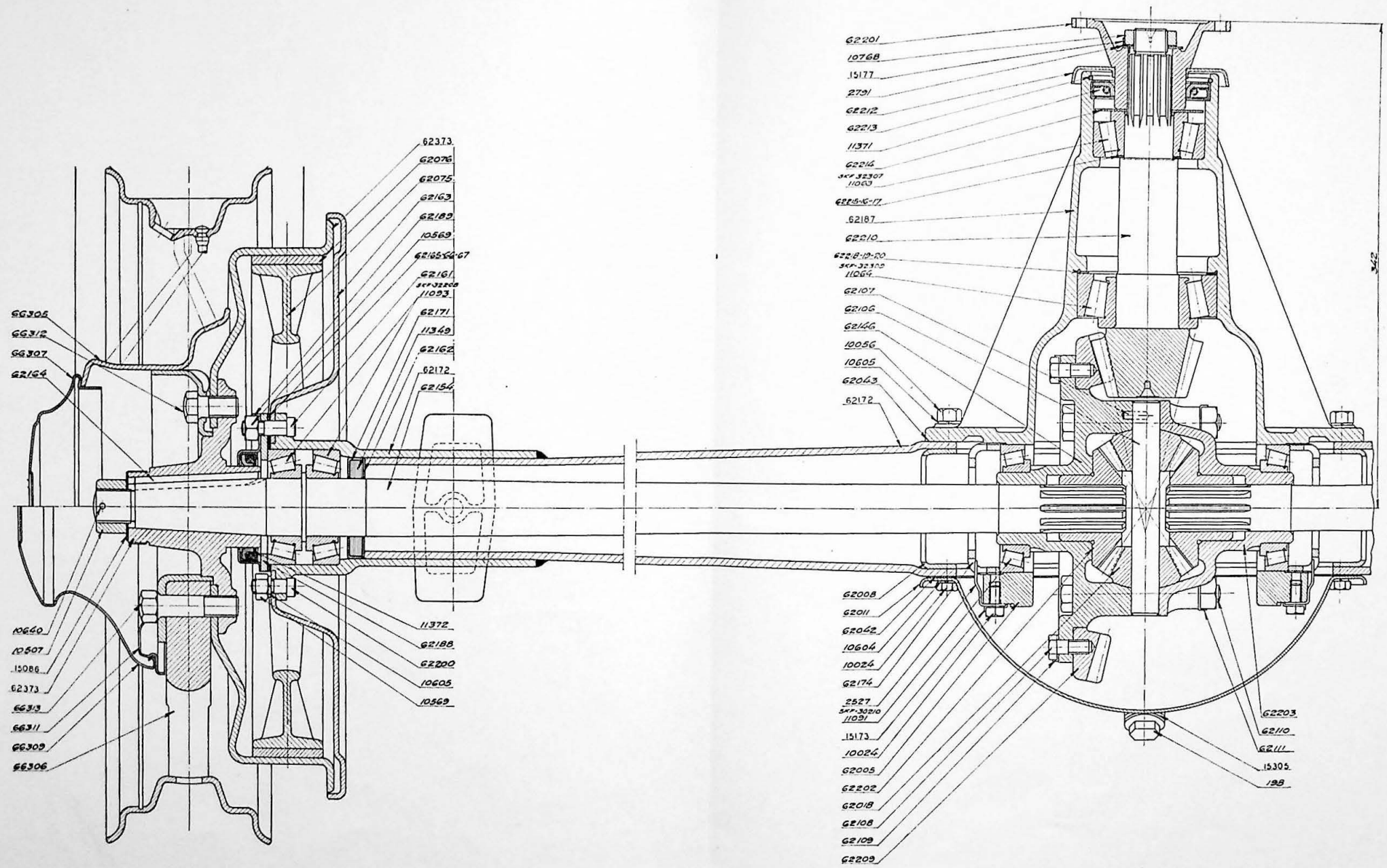
Fig. 179. Bakaxel med demonterbart hus för bakaxelväxel. (Bakaxelväxel, det. nr 62153).
