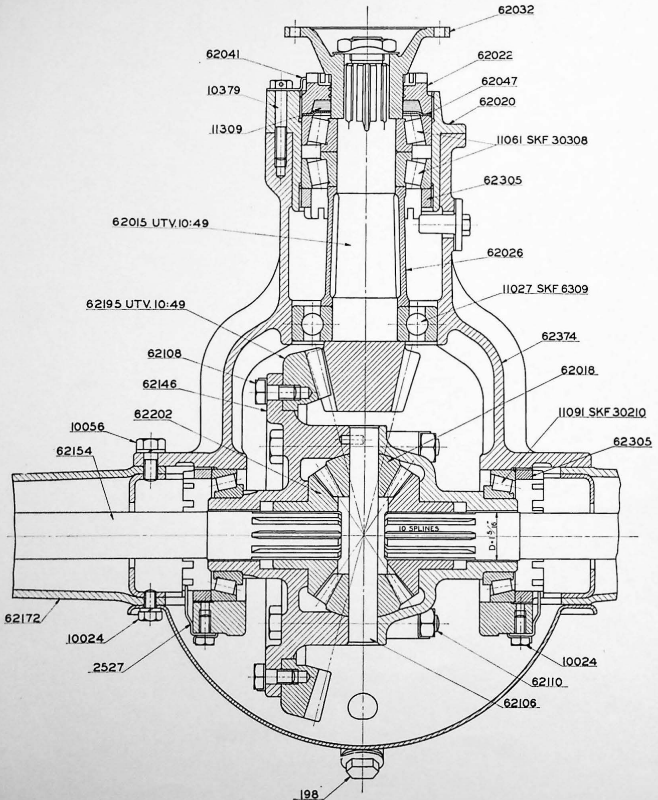
Fig. 180. Bakaxelväxel, det. nr 62266.
