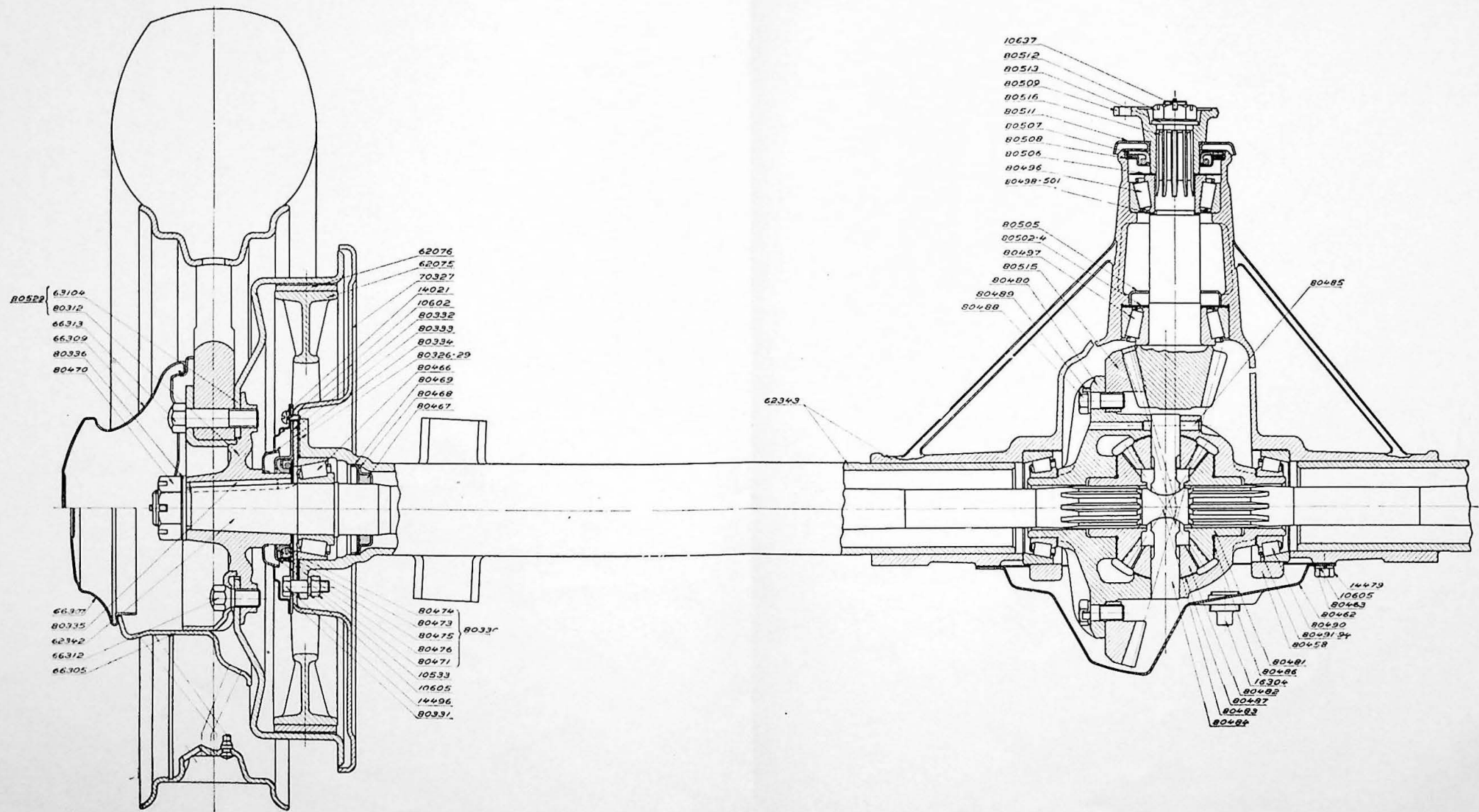
Fig. 181. Bakaxel, det. nr 62341.
