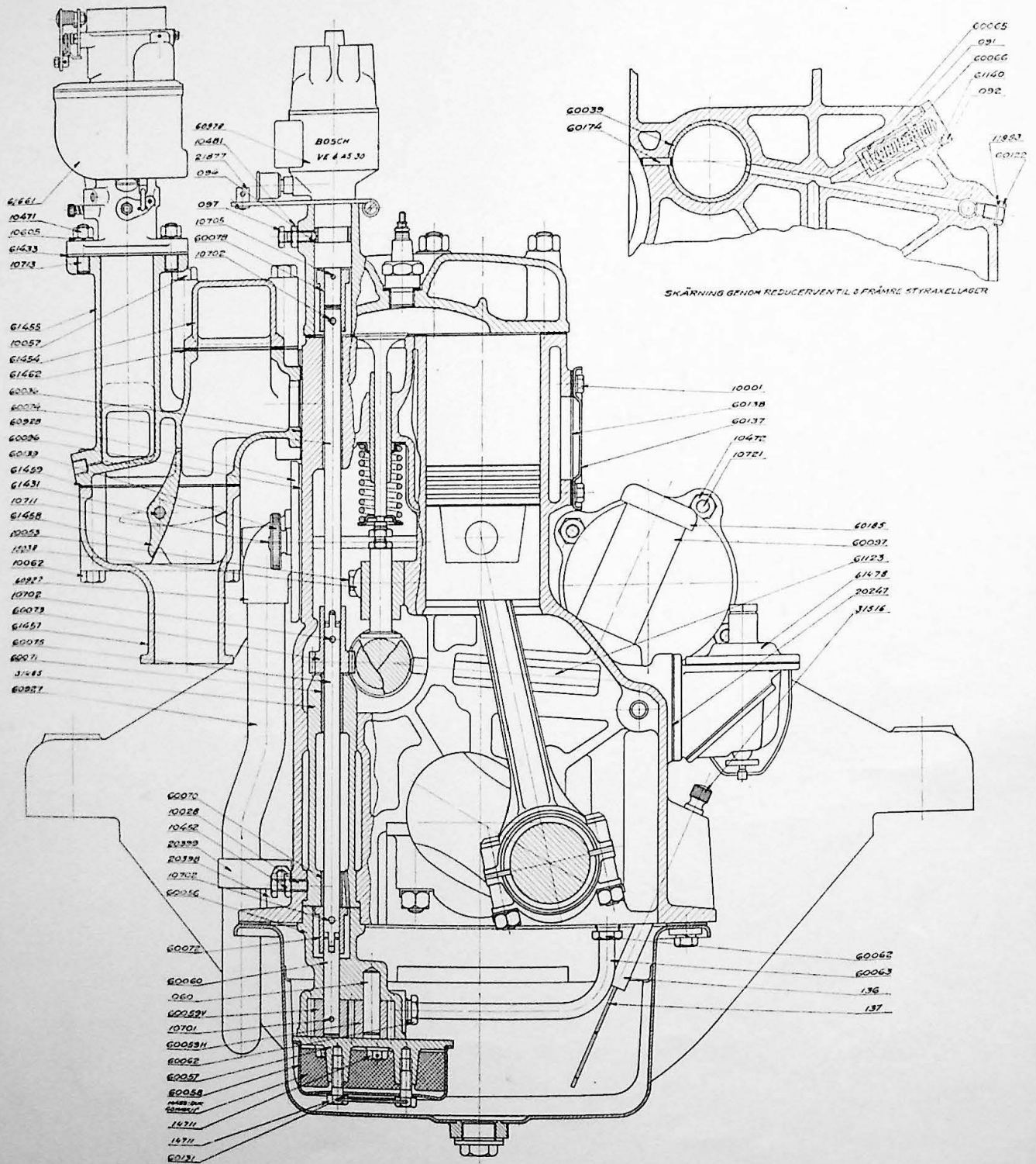
Fig. 173. Tvärsektion av EB-motor.
