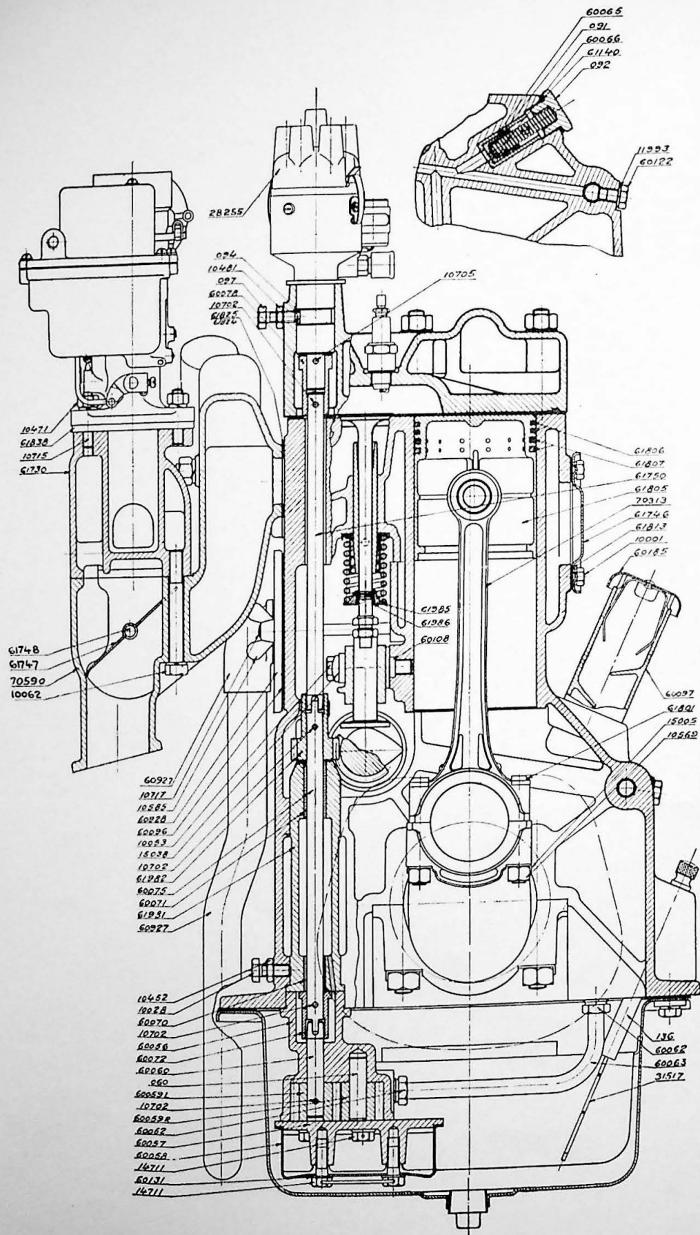
Fig. 175. Tvärsektion av EC-motor.
