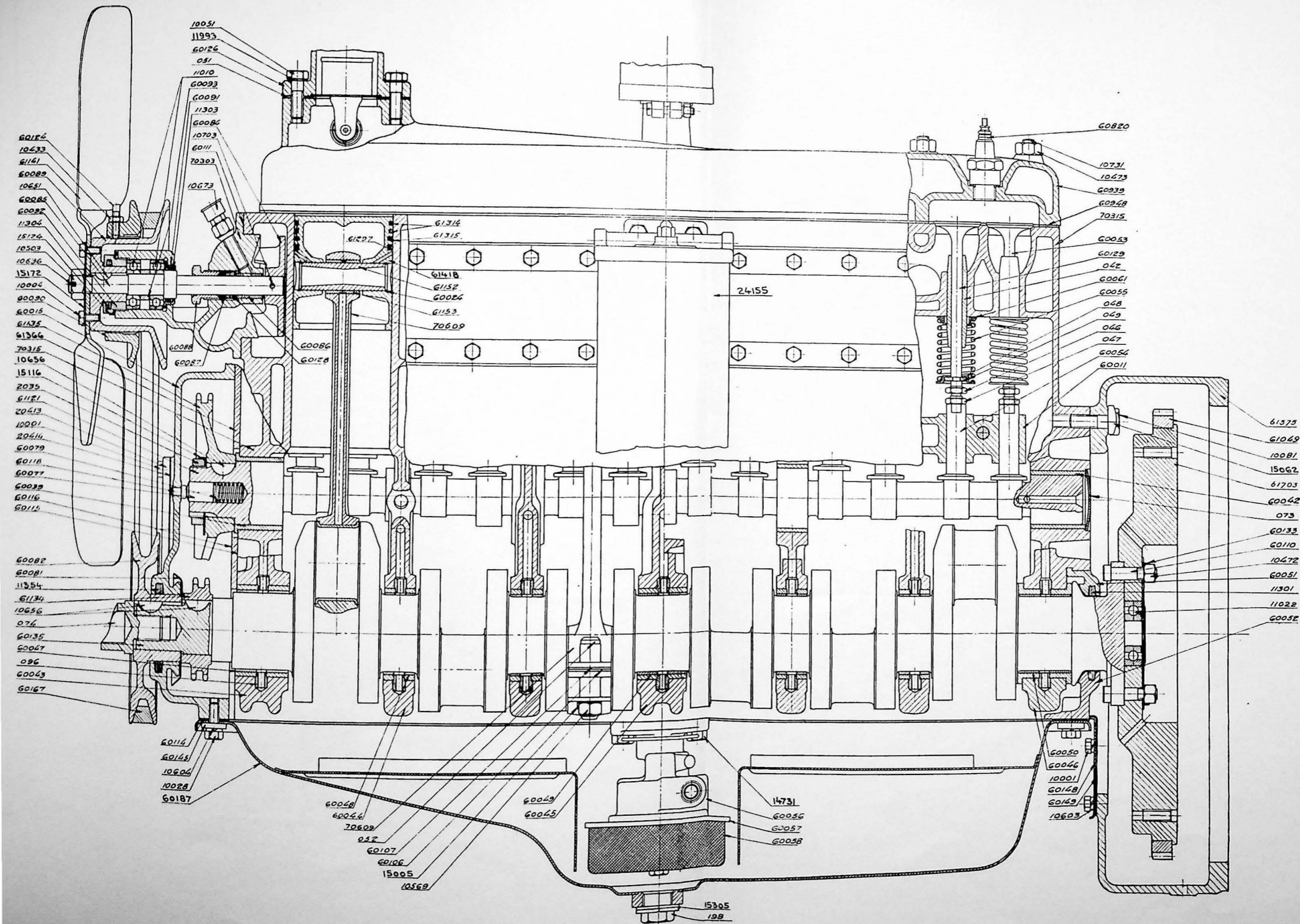
Fig. 172. Längdsektion av EB-motor.
