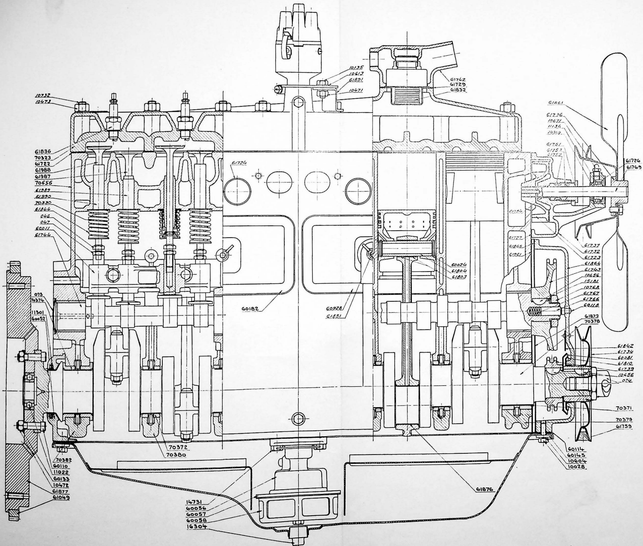
Fig. 174. Längdsektion av EC-motor.
