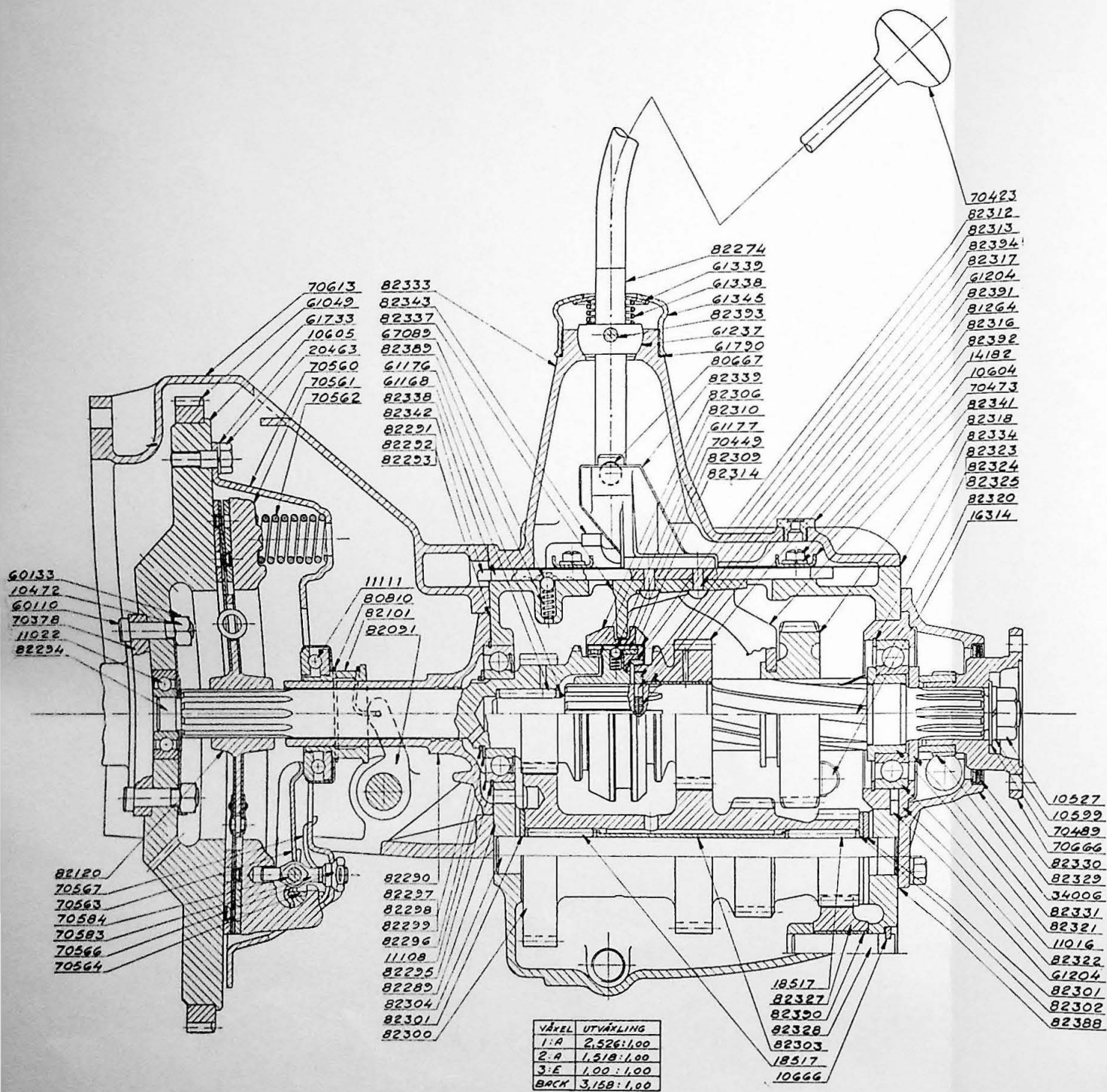
Plansch II. Sektion av koppling och växellåda.
