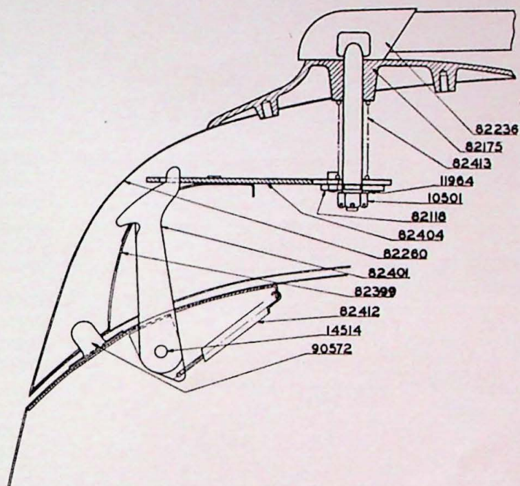
Fig. 29. Låsanordning för motorhuv; tidigare utförande.
