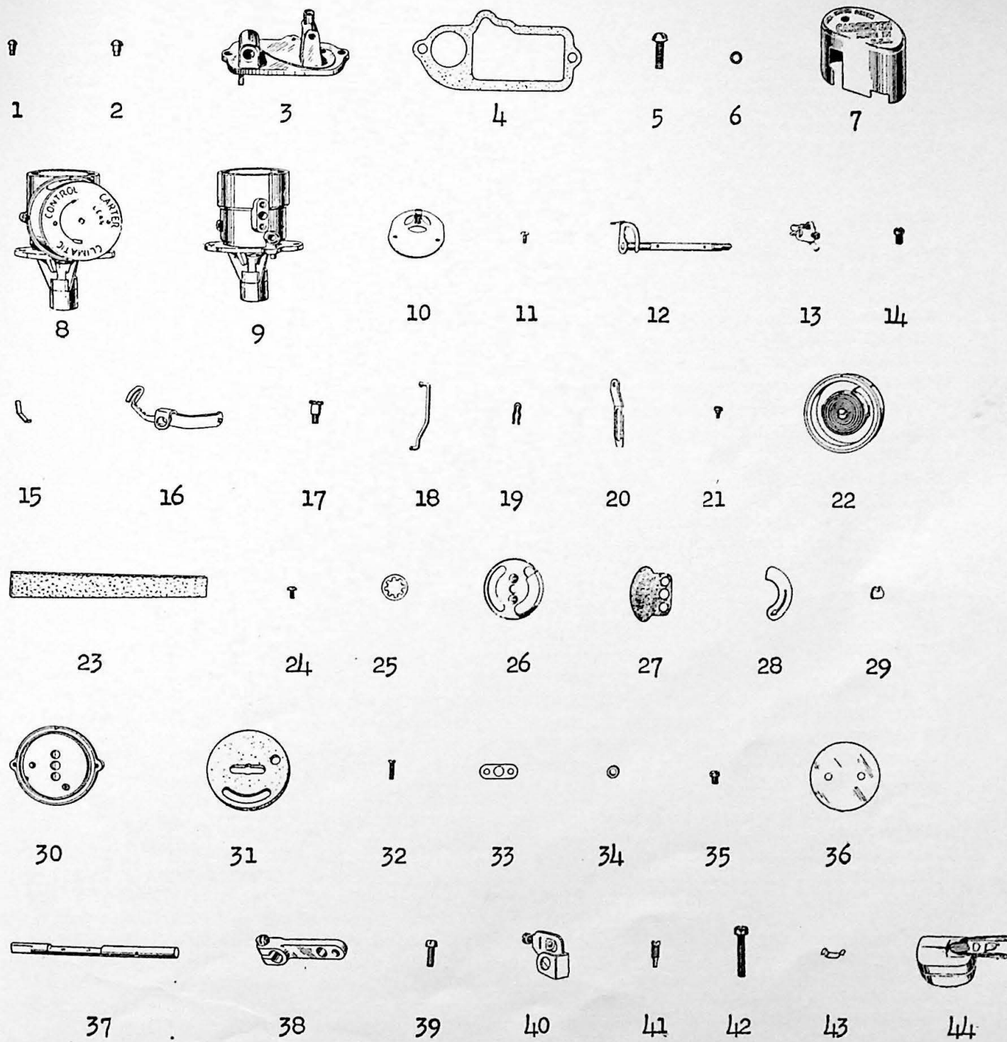
Fig. 16. Detaljer till förgasare.
