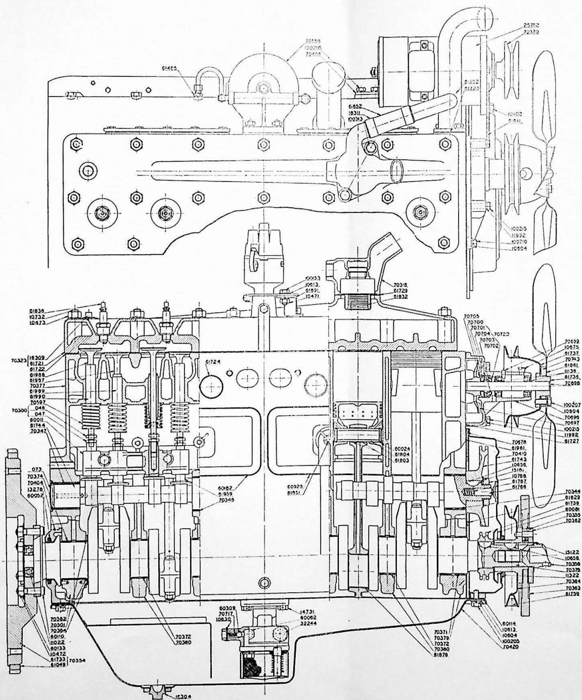
Plansch I. Sektion av EC-motor.
