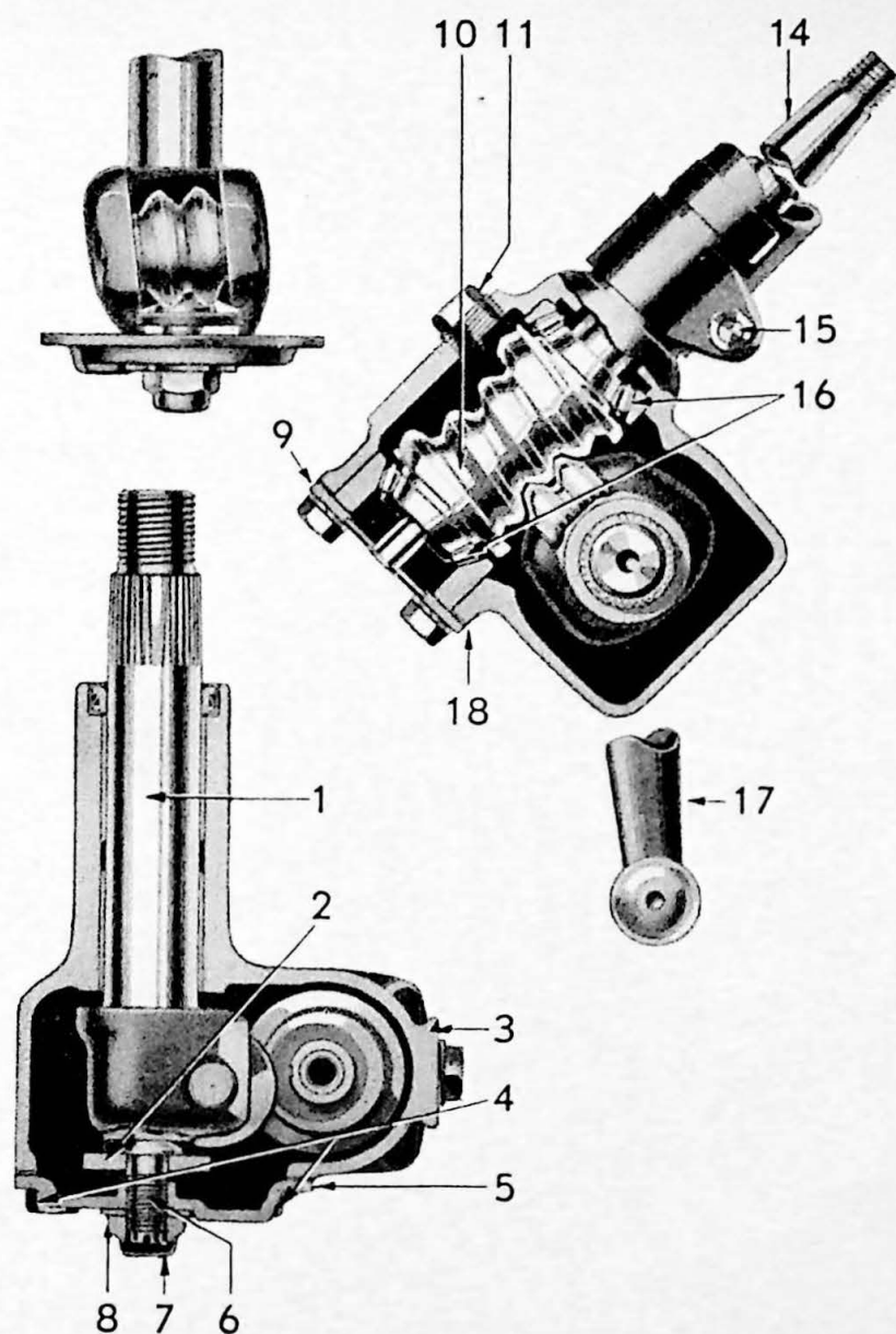
Fig. 27. Detaljer för styrinrättning.
